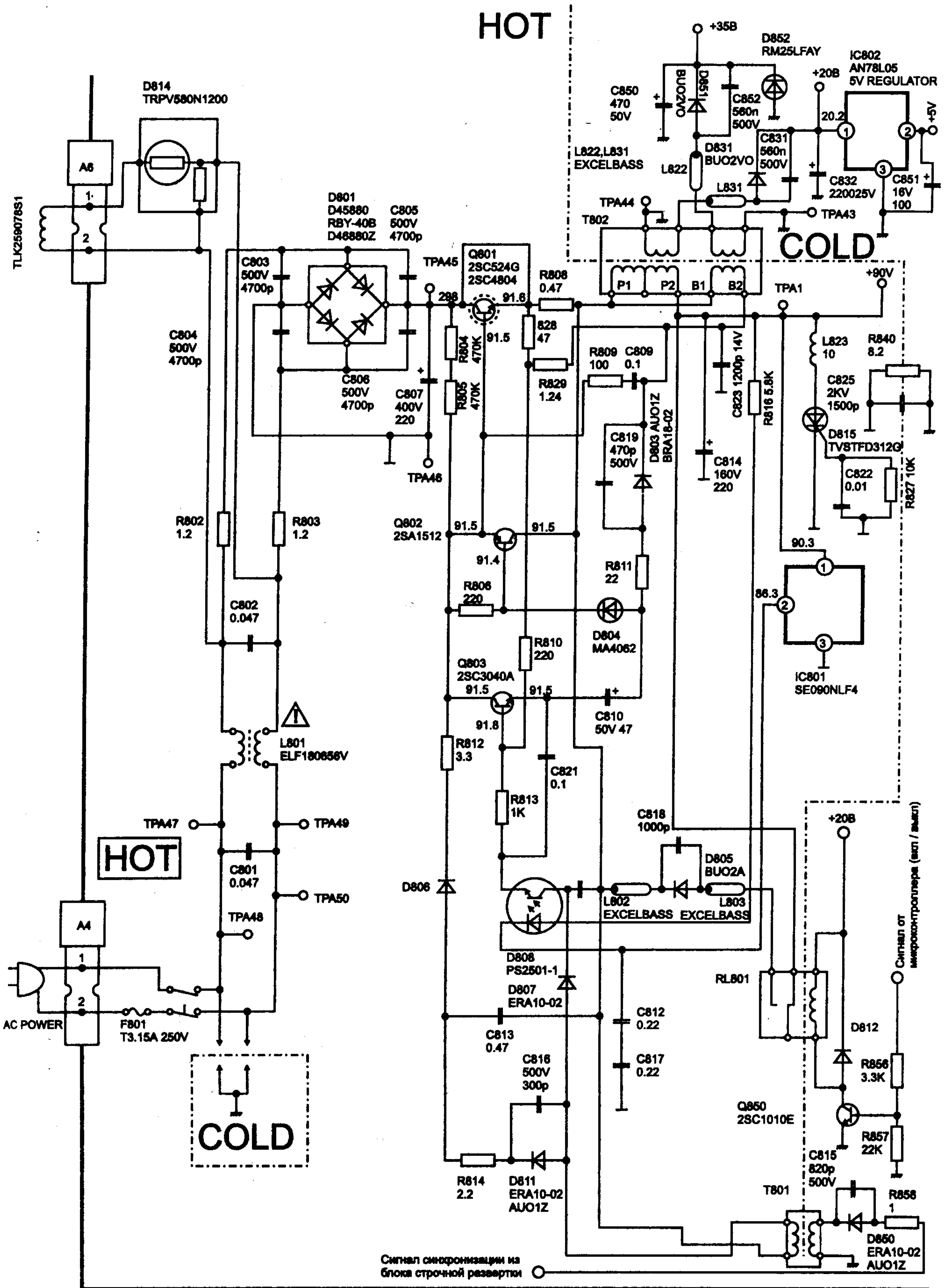
Принципиальная схема
