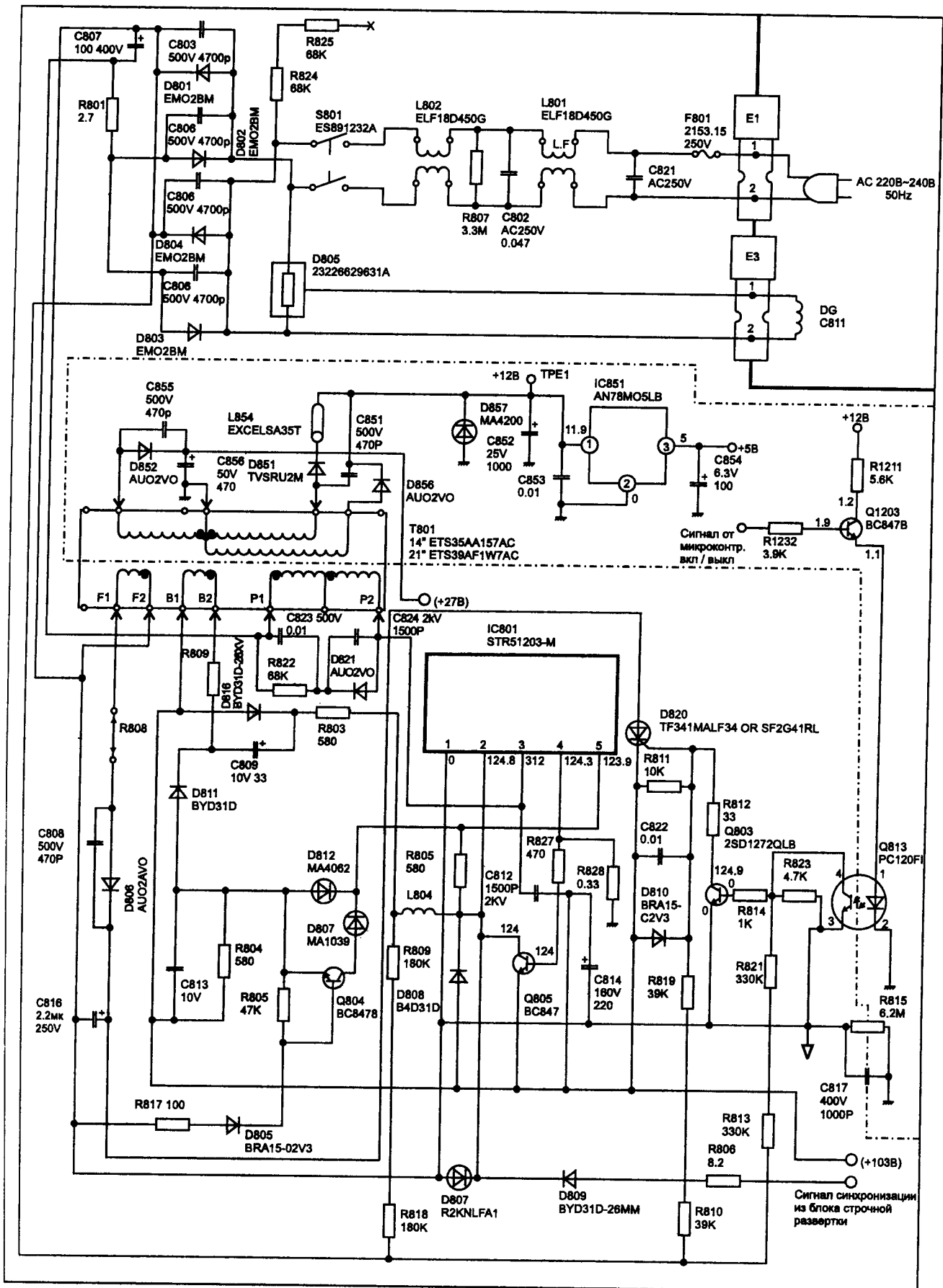
Принципиальная схема
