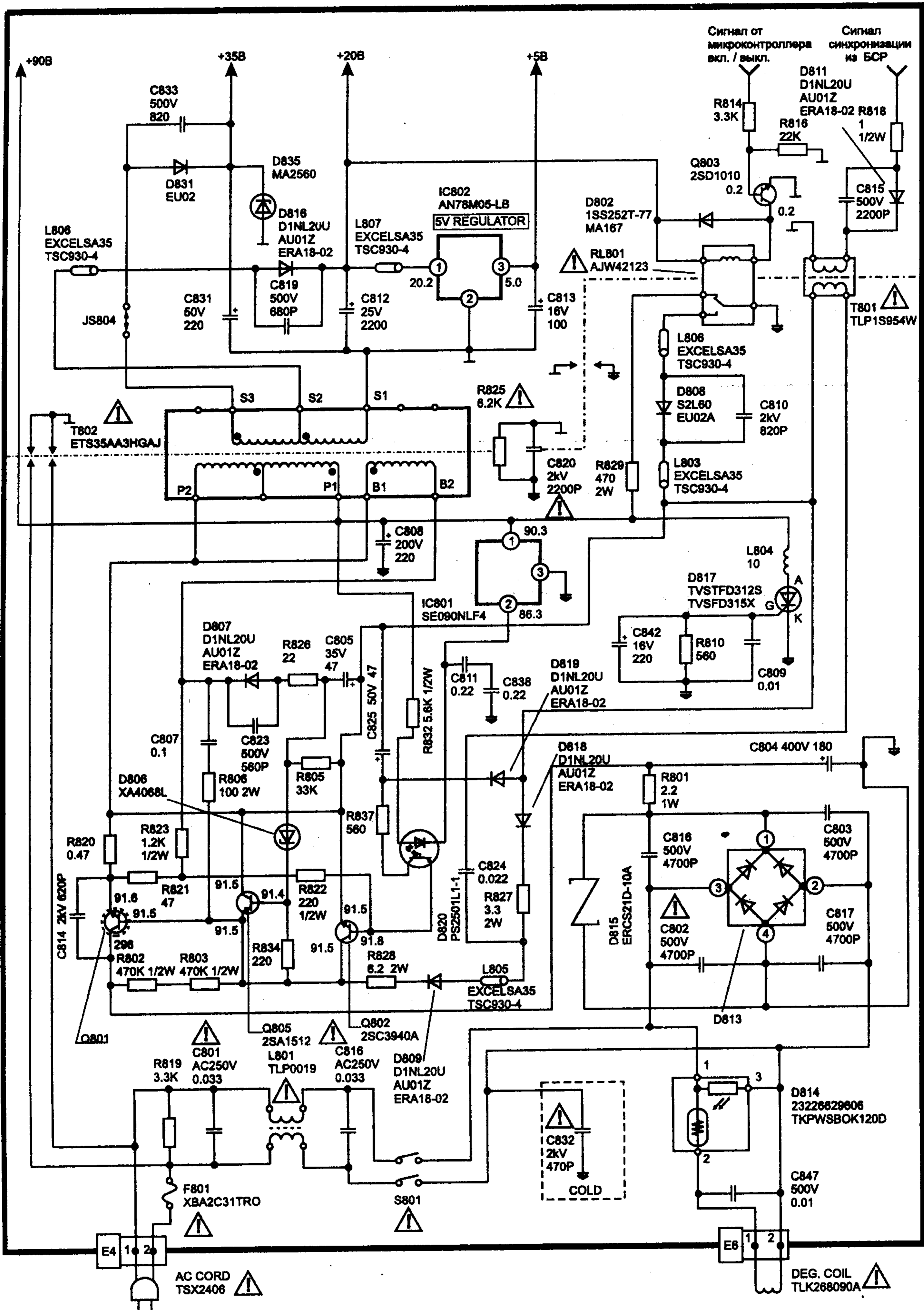
Схема блока питания телевизора PANASONIC TX-2170T, TC-2170R, TX-21F1T
