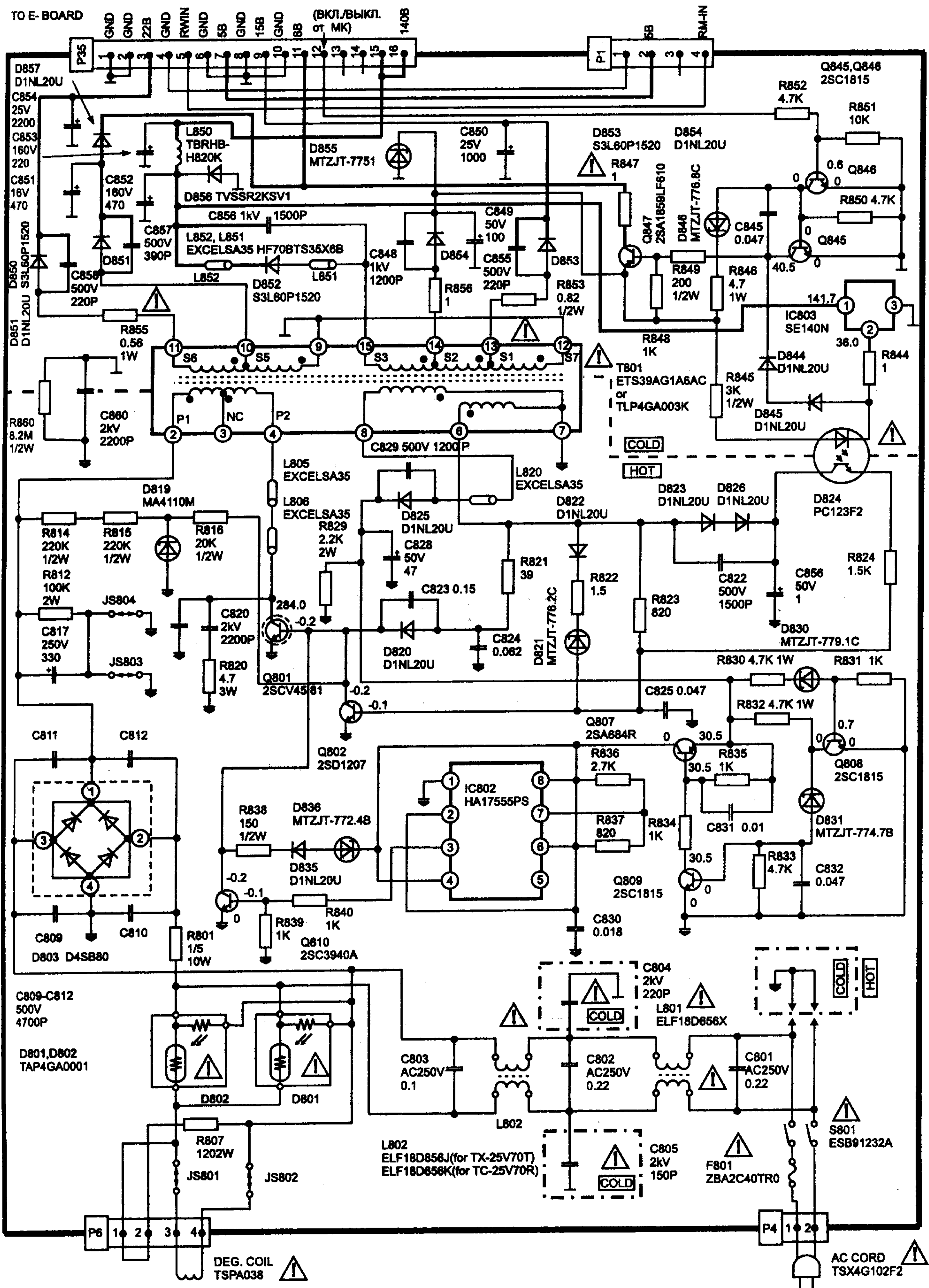
Принципиальная схема
