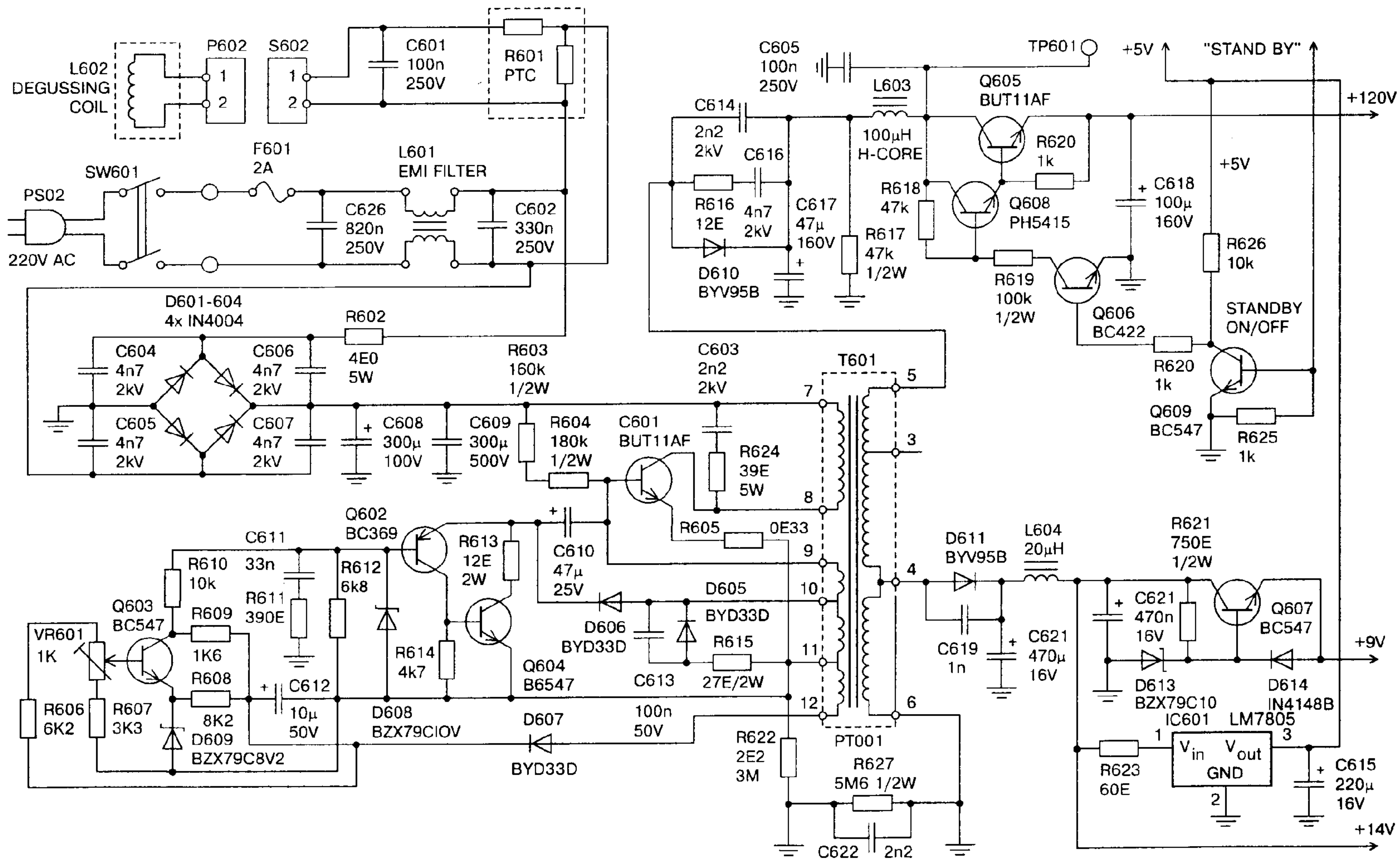
Схема блока питания телевизора RECOR 4020, 4021 Электрическая принципиальная схема источника TV «RECOR 4020/4021»
