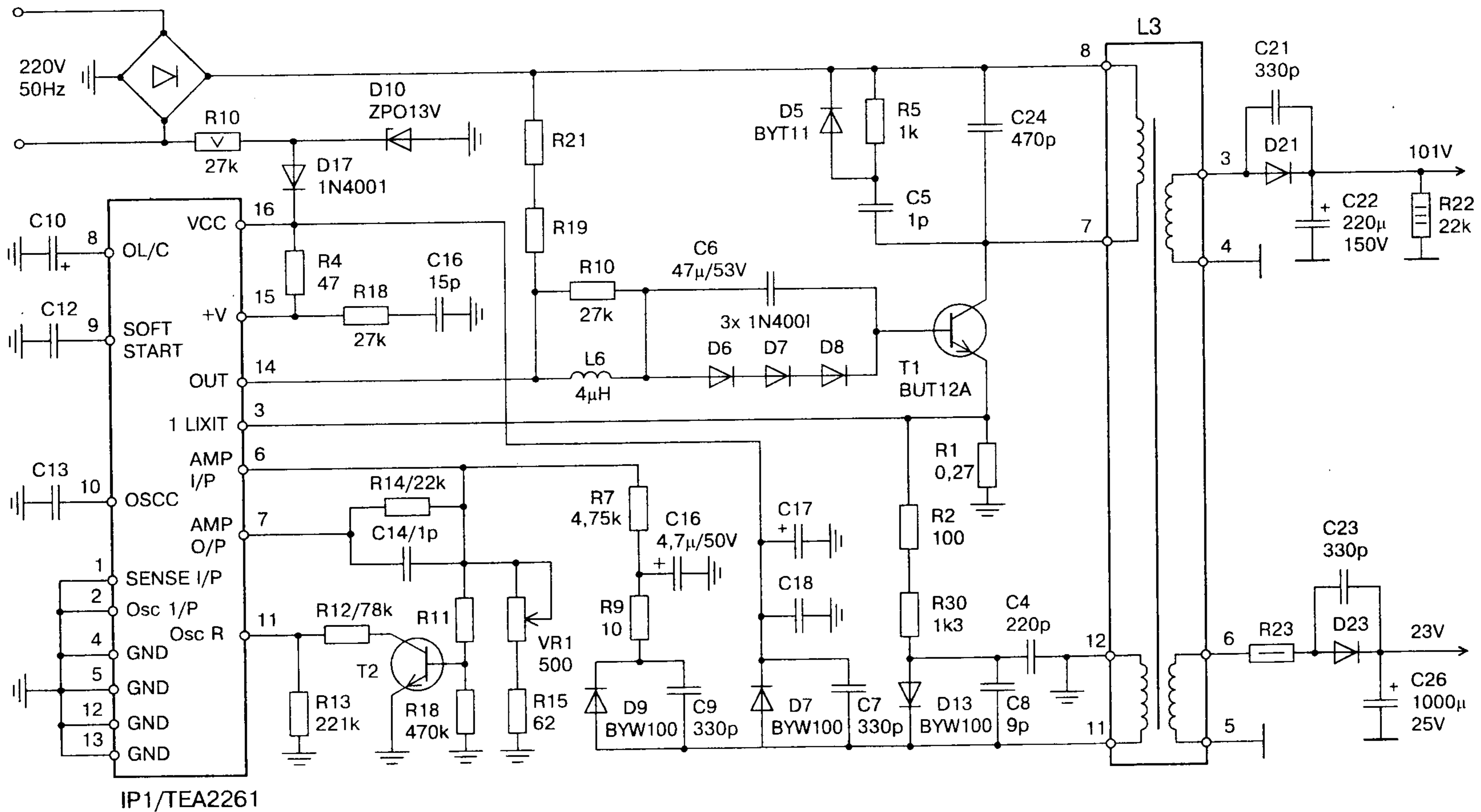
Схема блока питания телевизора SABA
