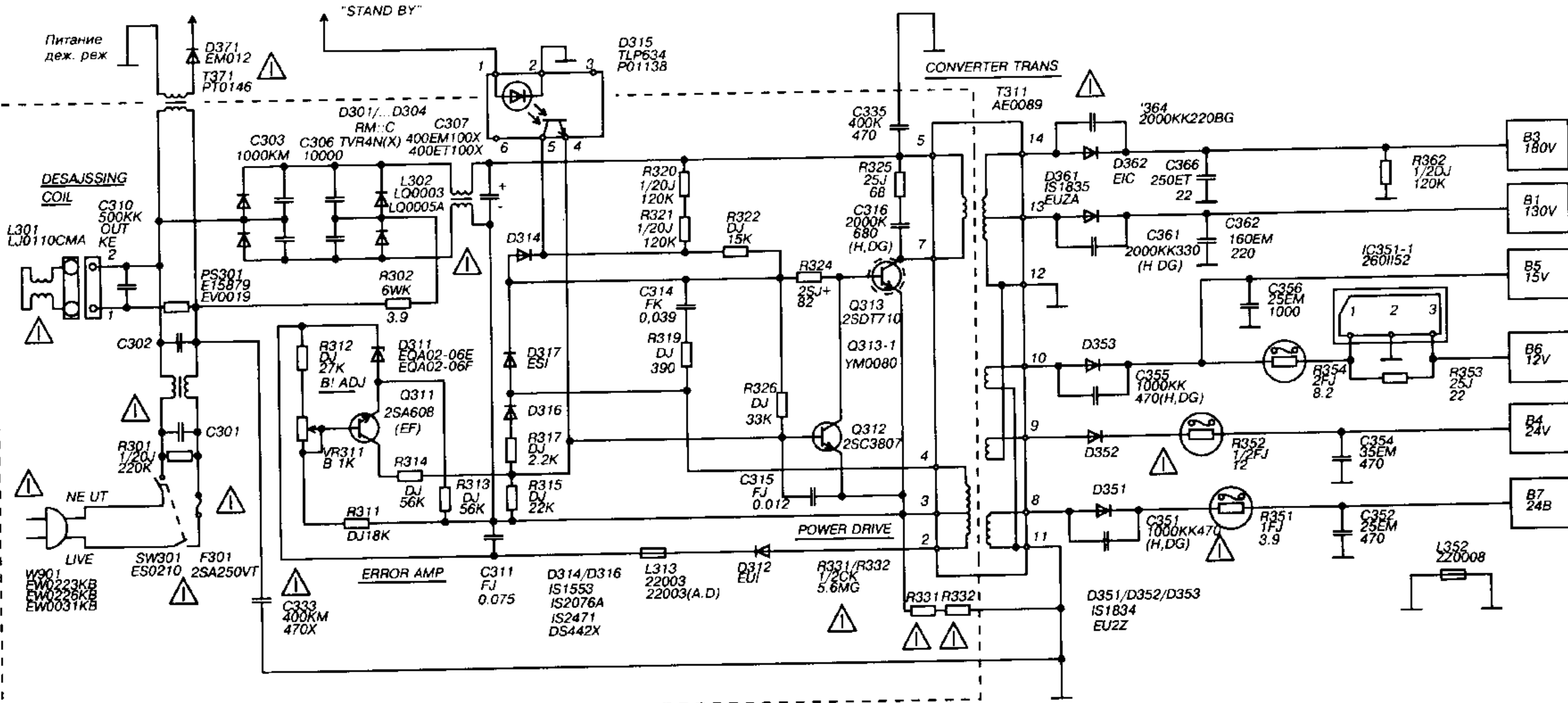
Схема блока питания телевизора SANYO CEM-2130 PV-20
