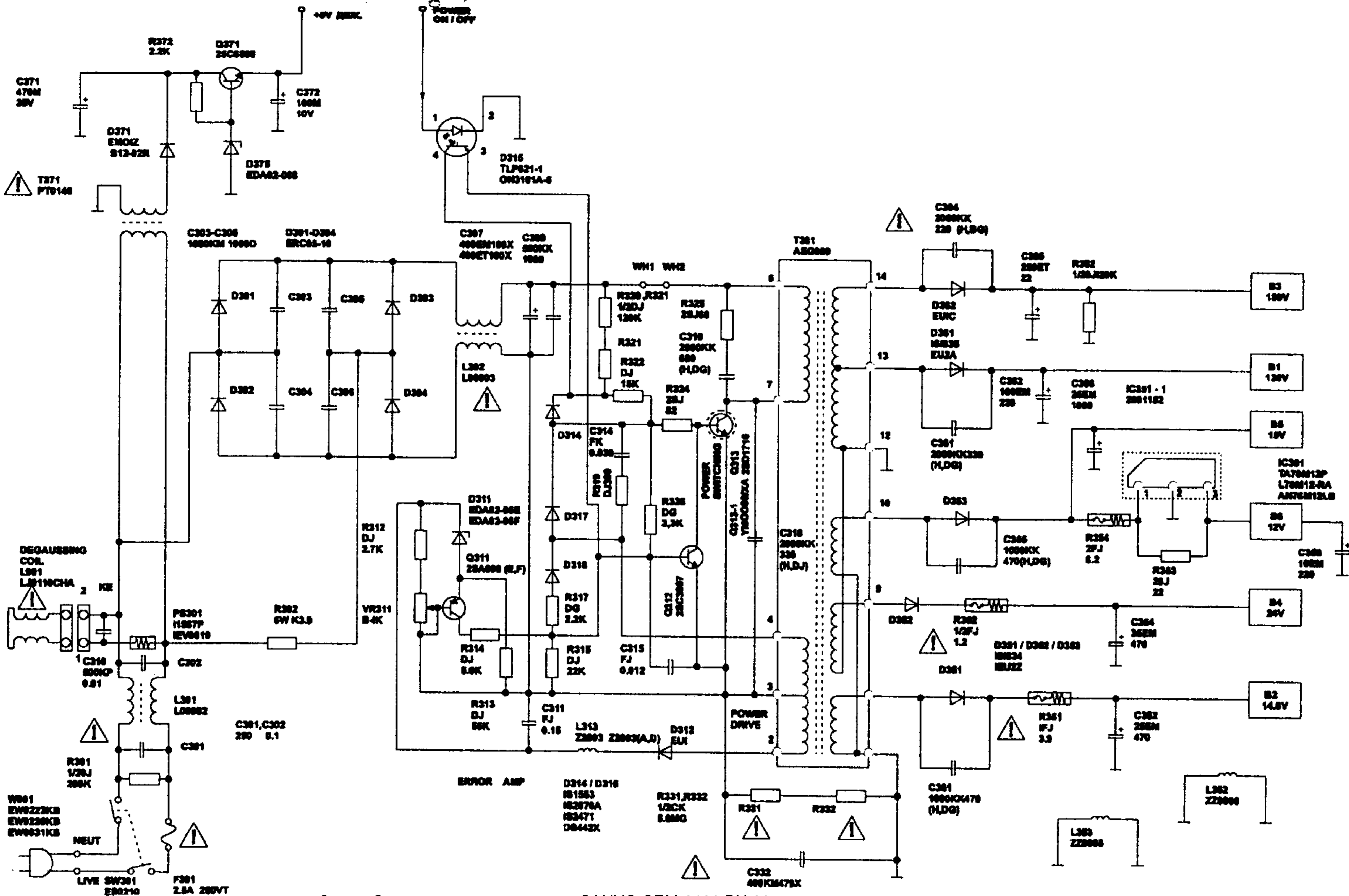
Схема блока питания телевизора SANYO CEM-2130 PX-20
