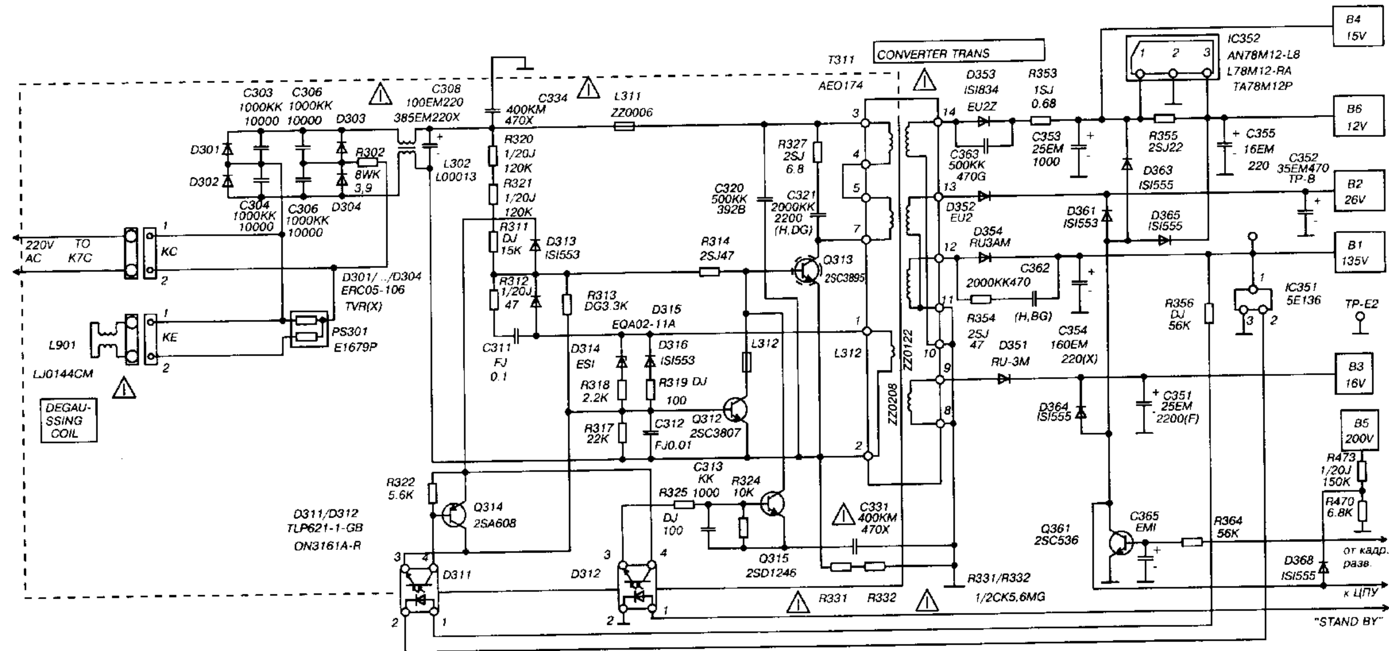
Схема блока питания телевизора SANYO CEM-2511 VCU-00 Схема электрическая принципиальная источника питания телевизора "SANYO CEM 2511 VSU-00"
