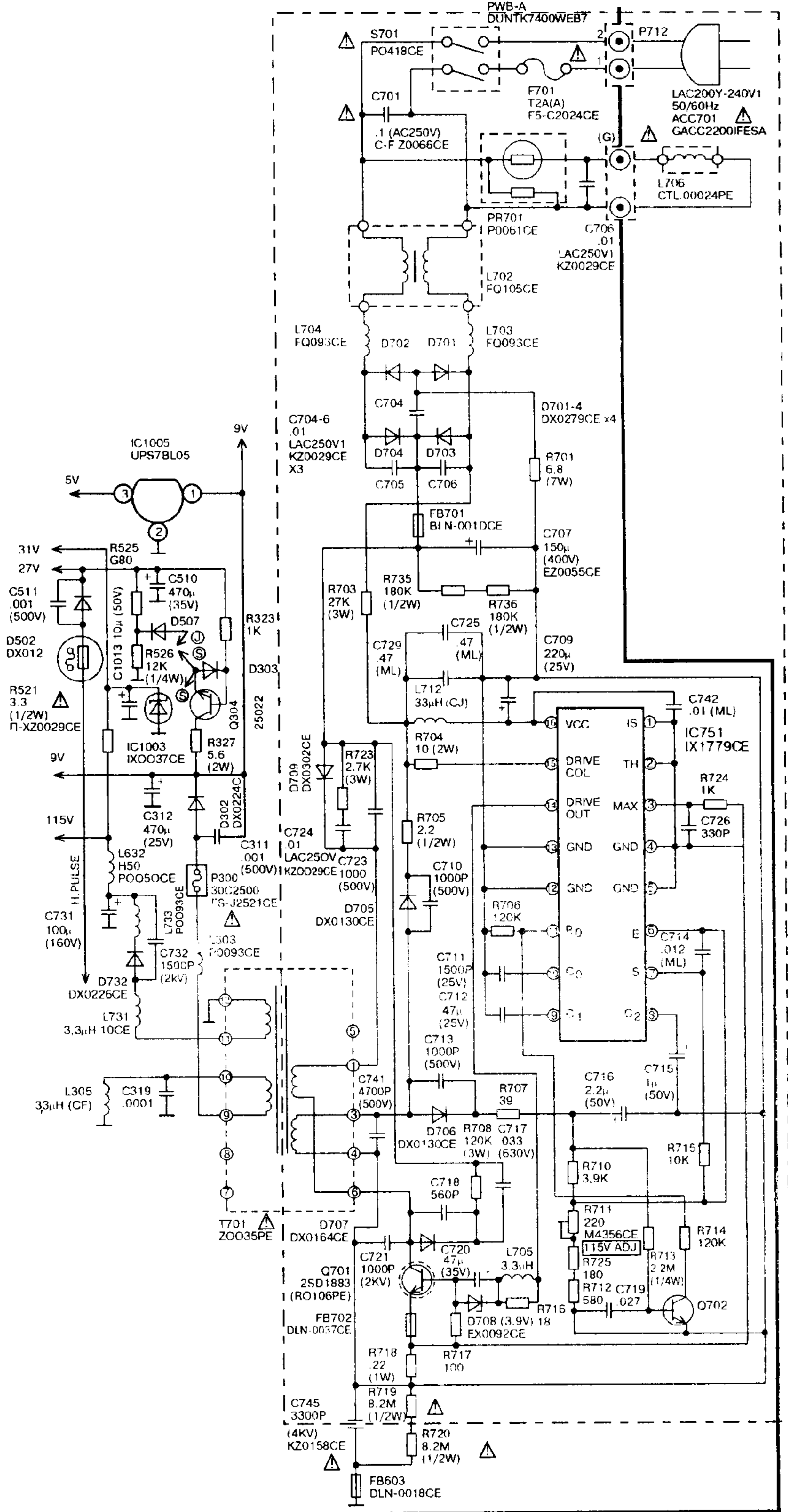
Схема блока питания телевизора SHARP 20B-SC Электрическая принципиальная схема источника SHARP 20B-SC
