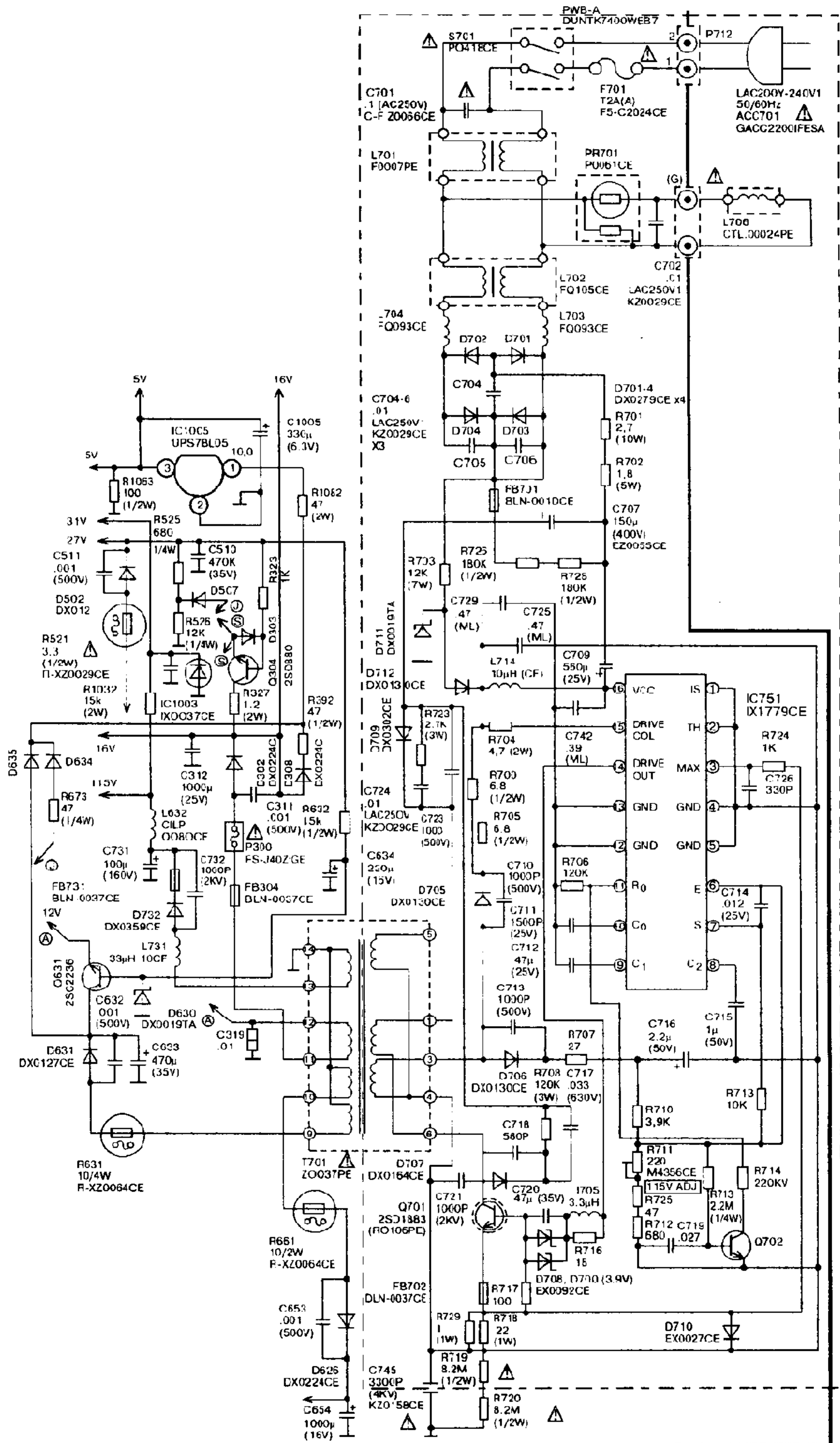
Схема блока питания телевизора SHARP 21B-N21
