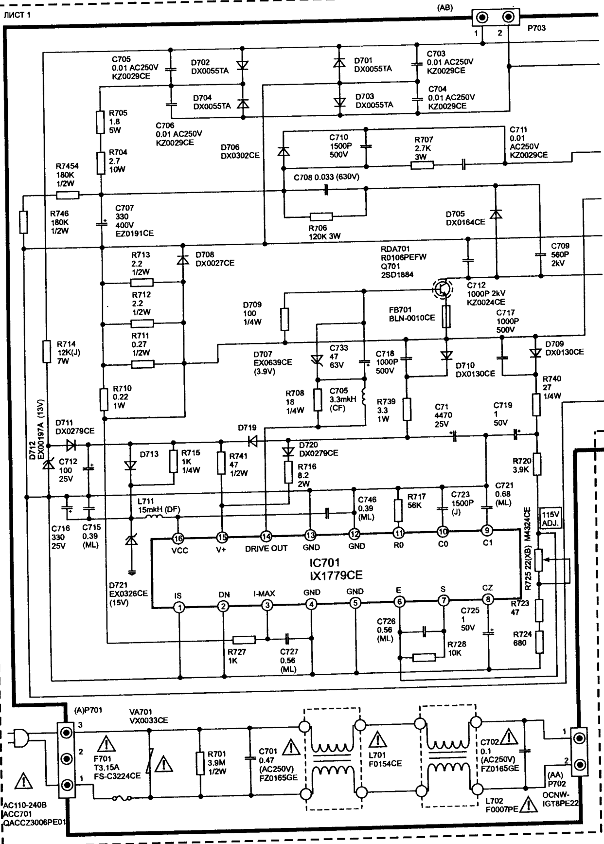
Принципиальная схема
