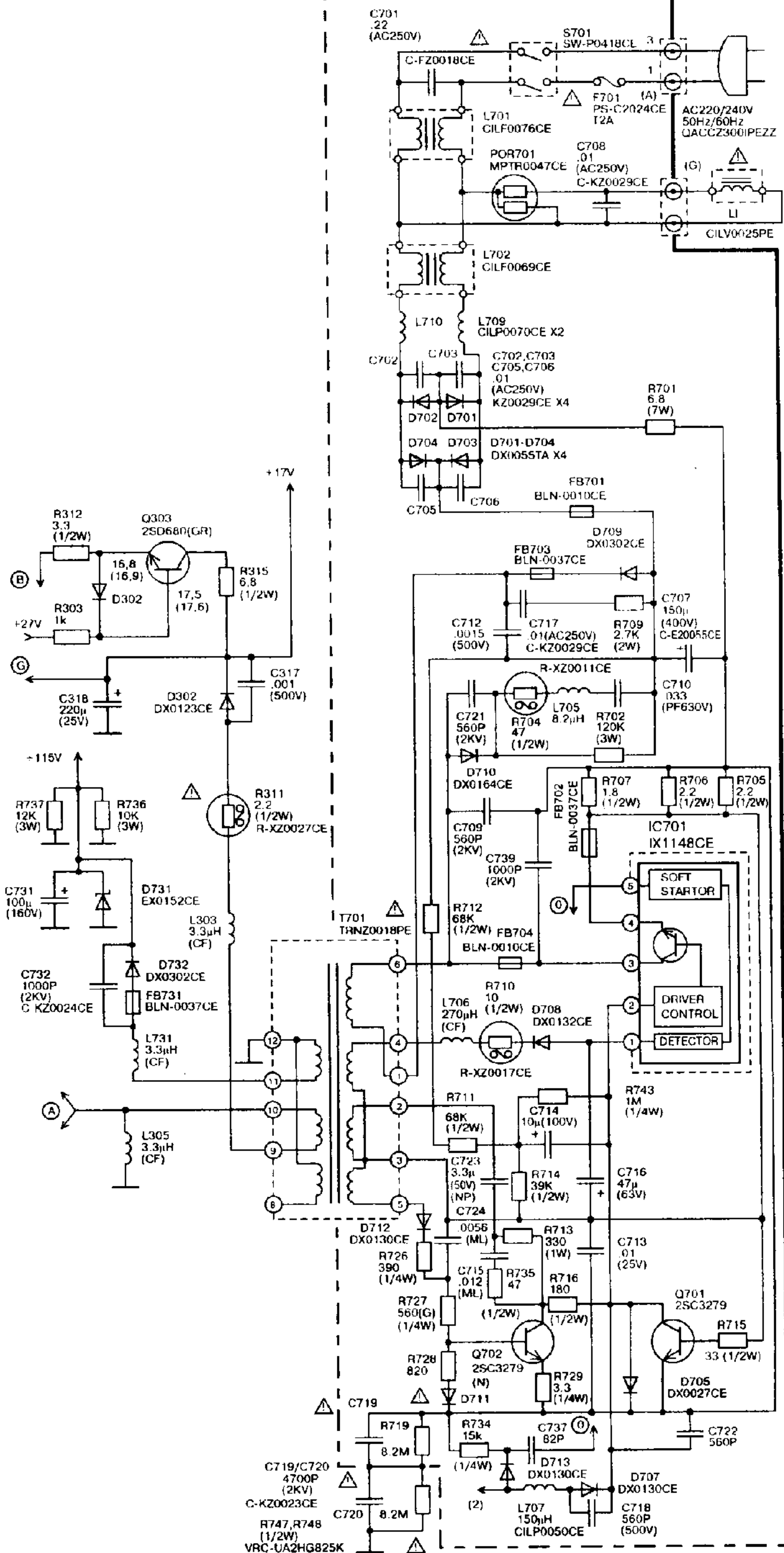
Схема блока питания телевизора SHARP SV-2131SK1
