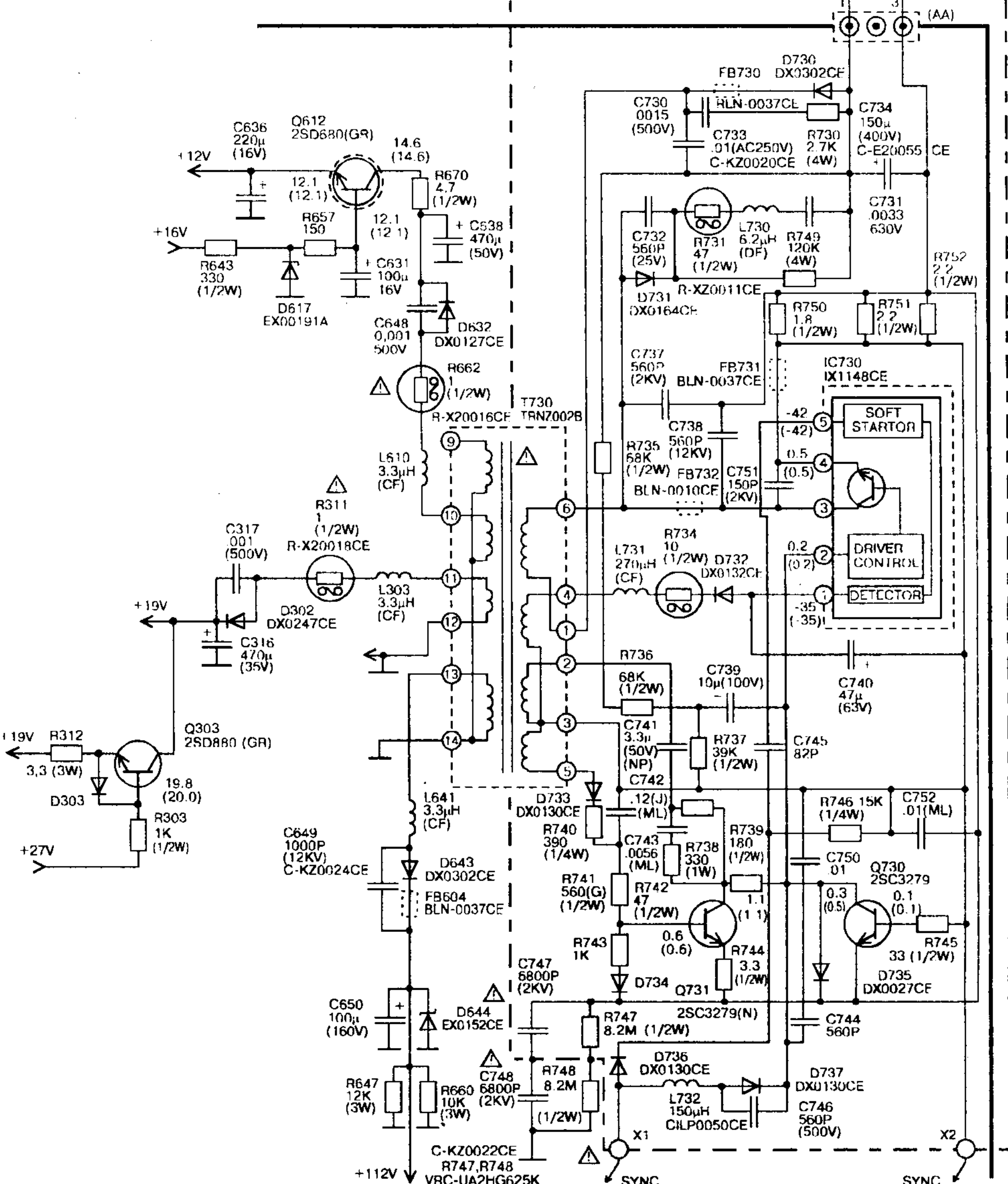
Схема блока питания телевизора SHARP SV-2142S
