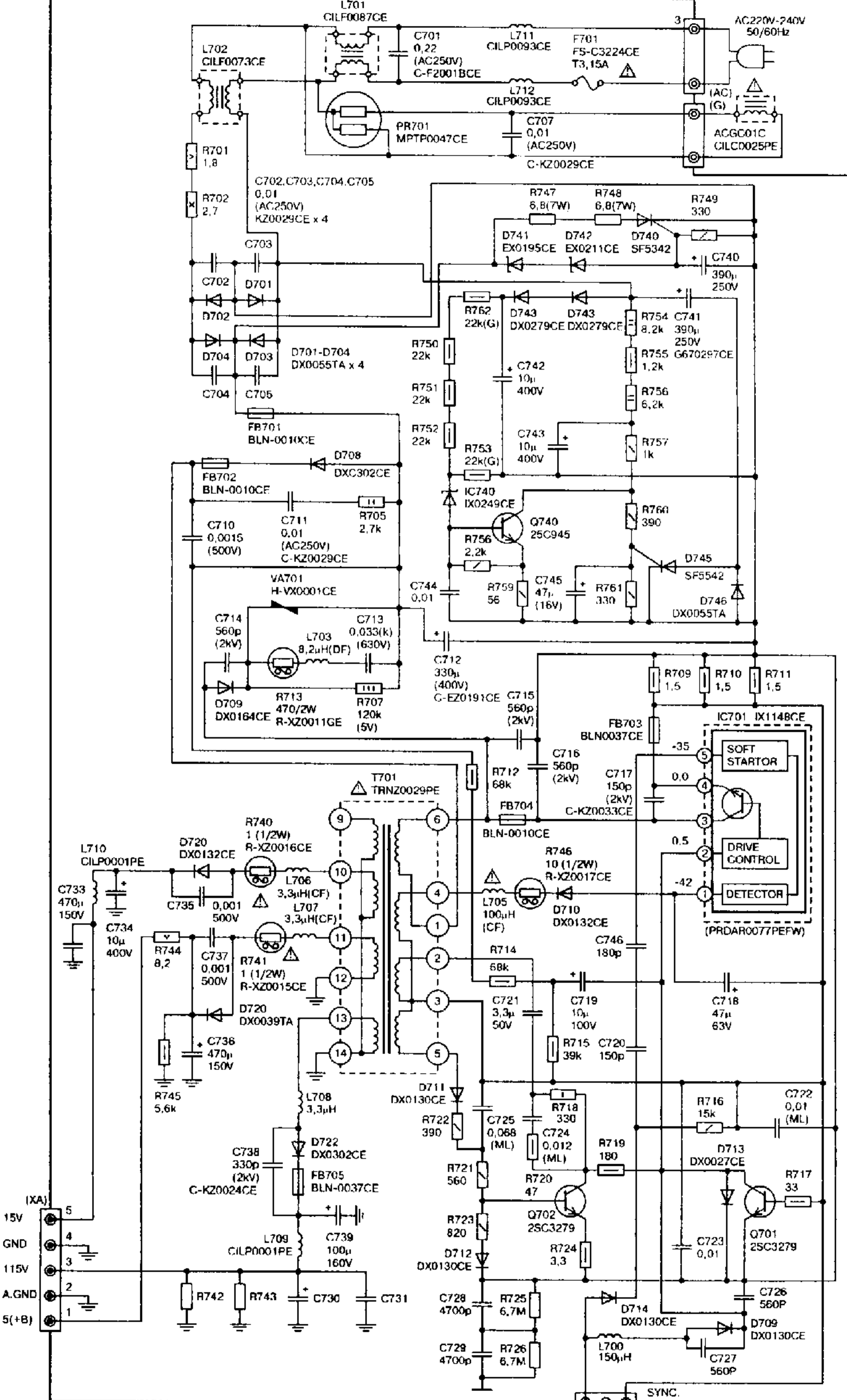
Схема блока питания телевизора SHARP SV-2152U
