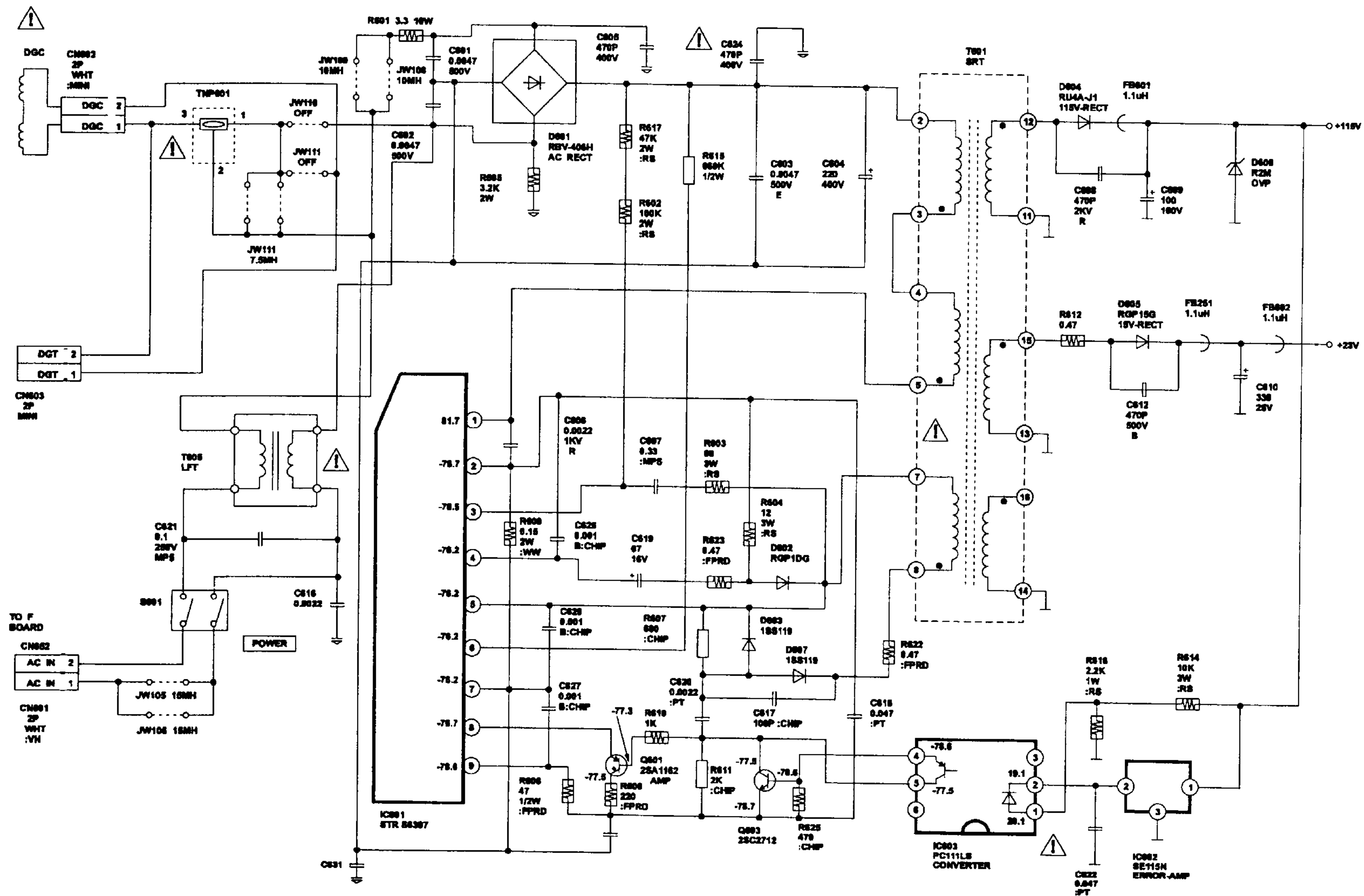
Схема блока питания телевизора SONY KV-1485MT
