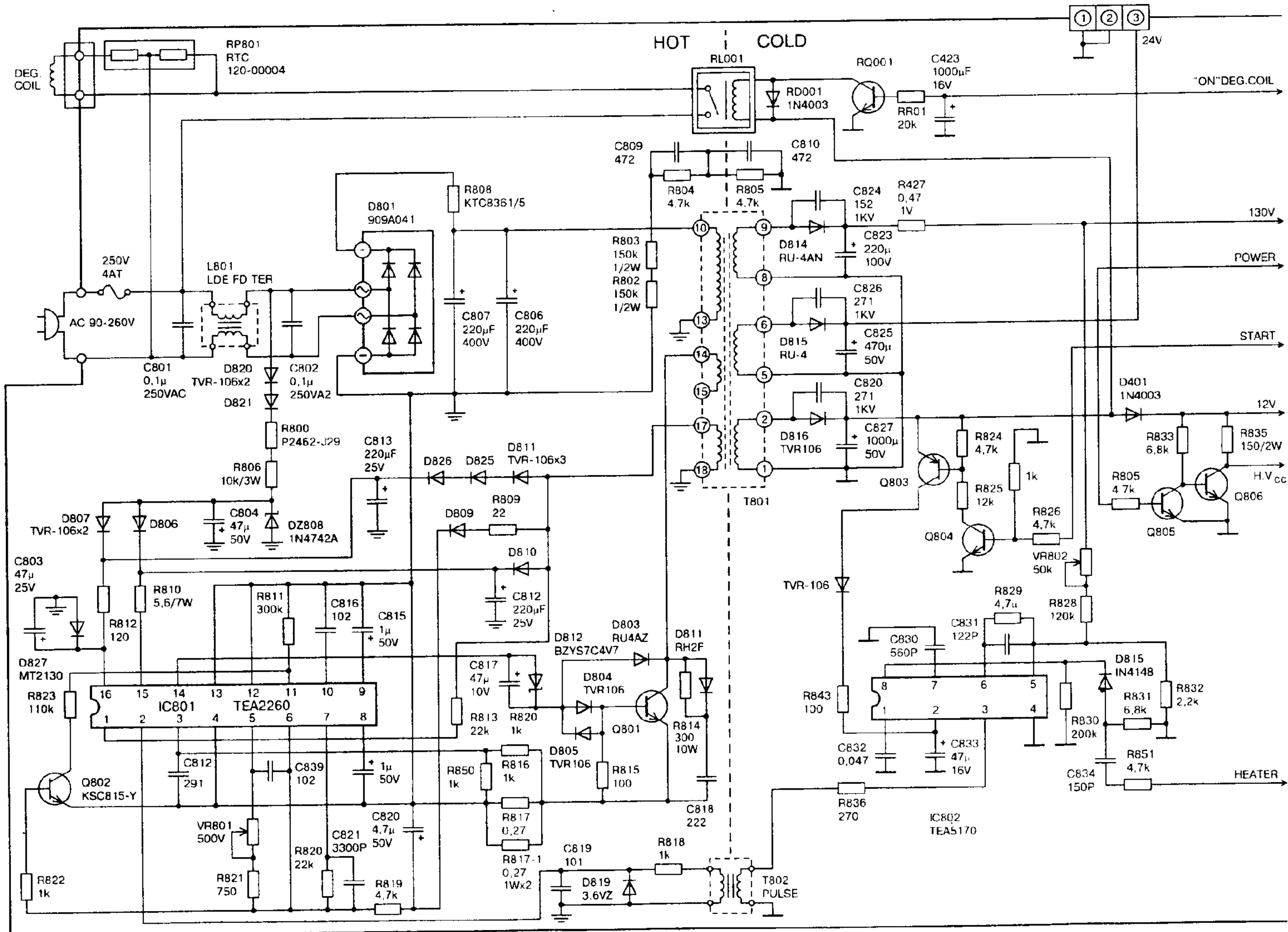
Схема блока питания телевизора SUPRA STV-2910MS
