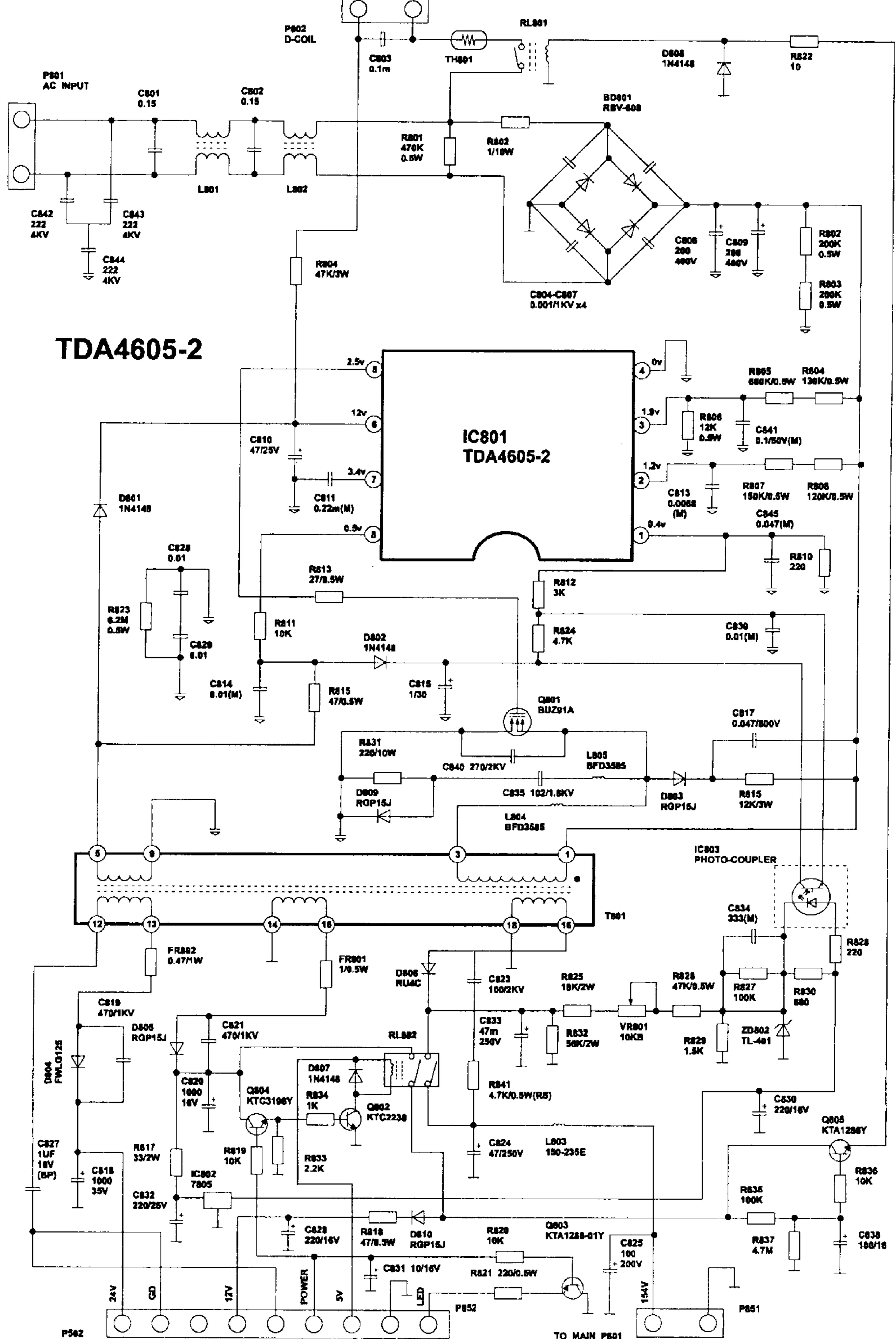
Схема блока питания телевизора SUPRA STV-2924
