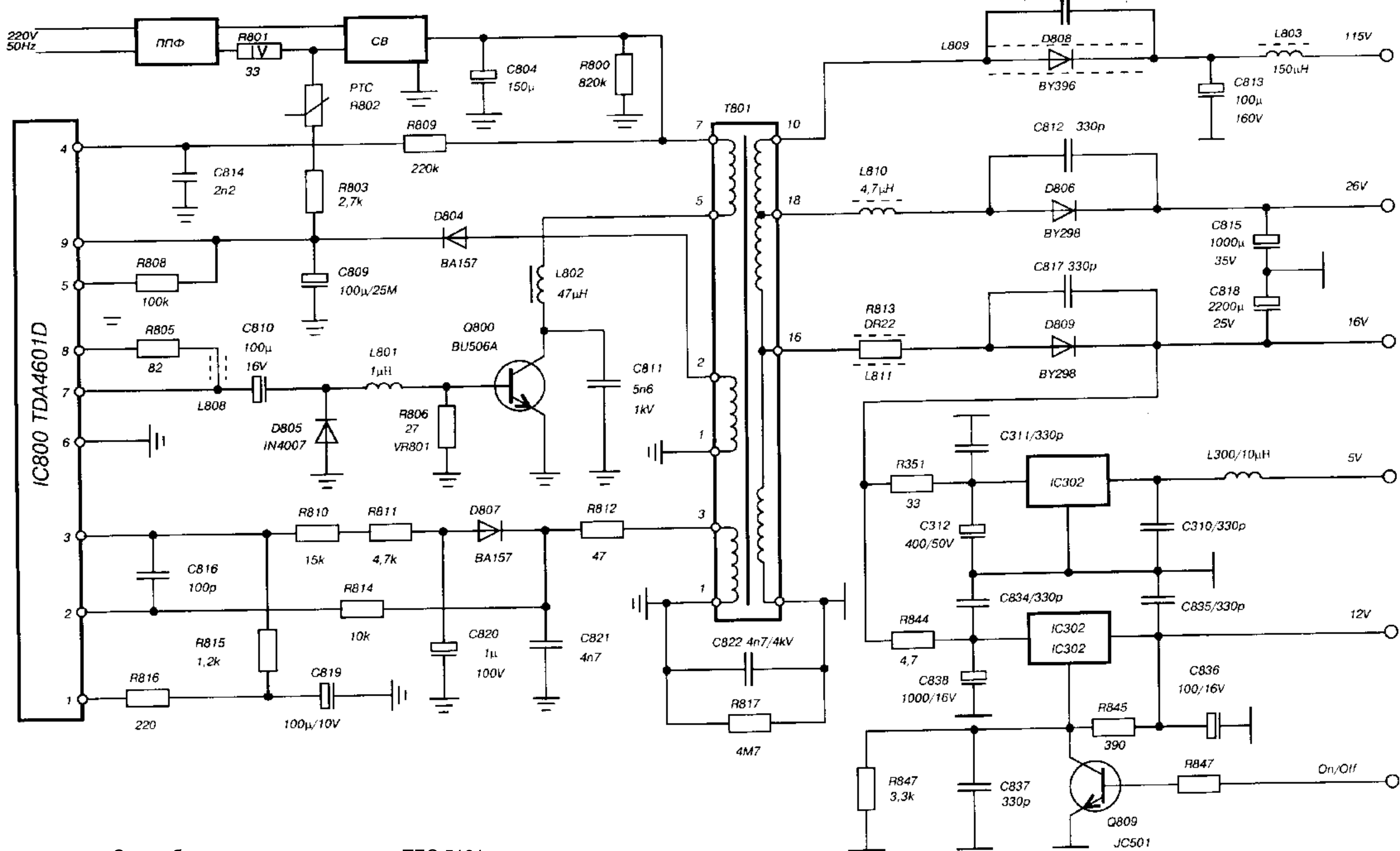
Схема блока питания телевизора ТЕС 5181
