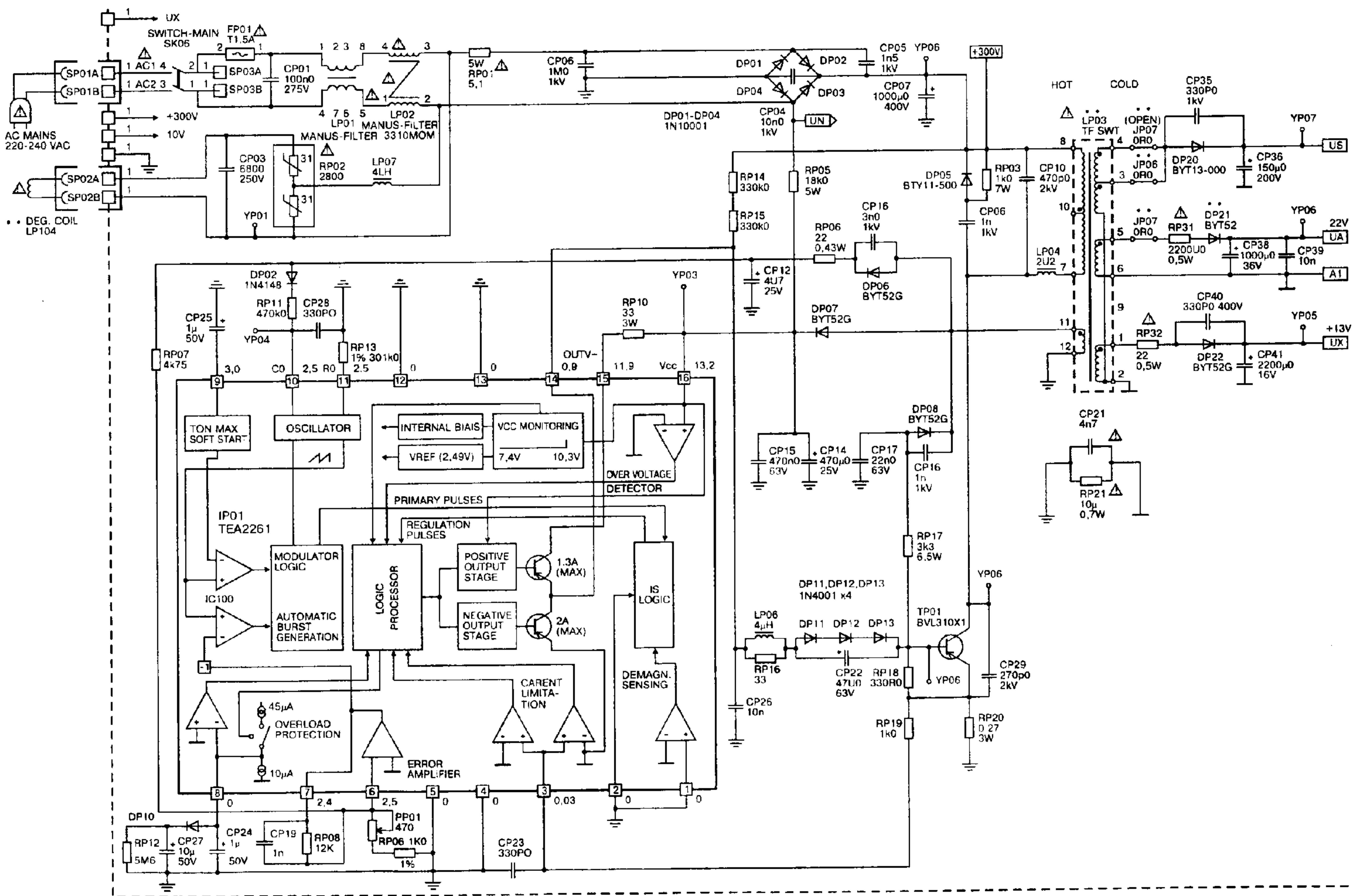
Схема блока питания телевизора THOMSON TX-91
