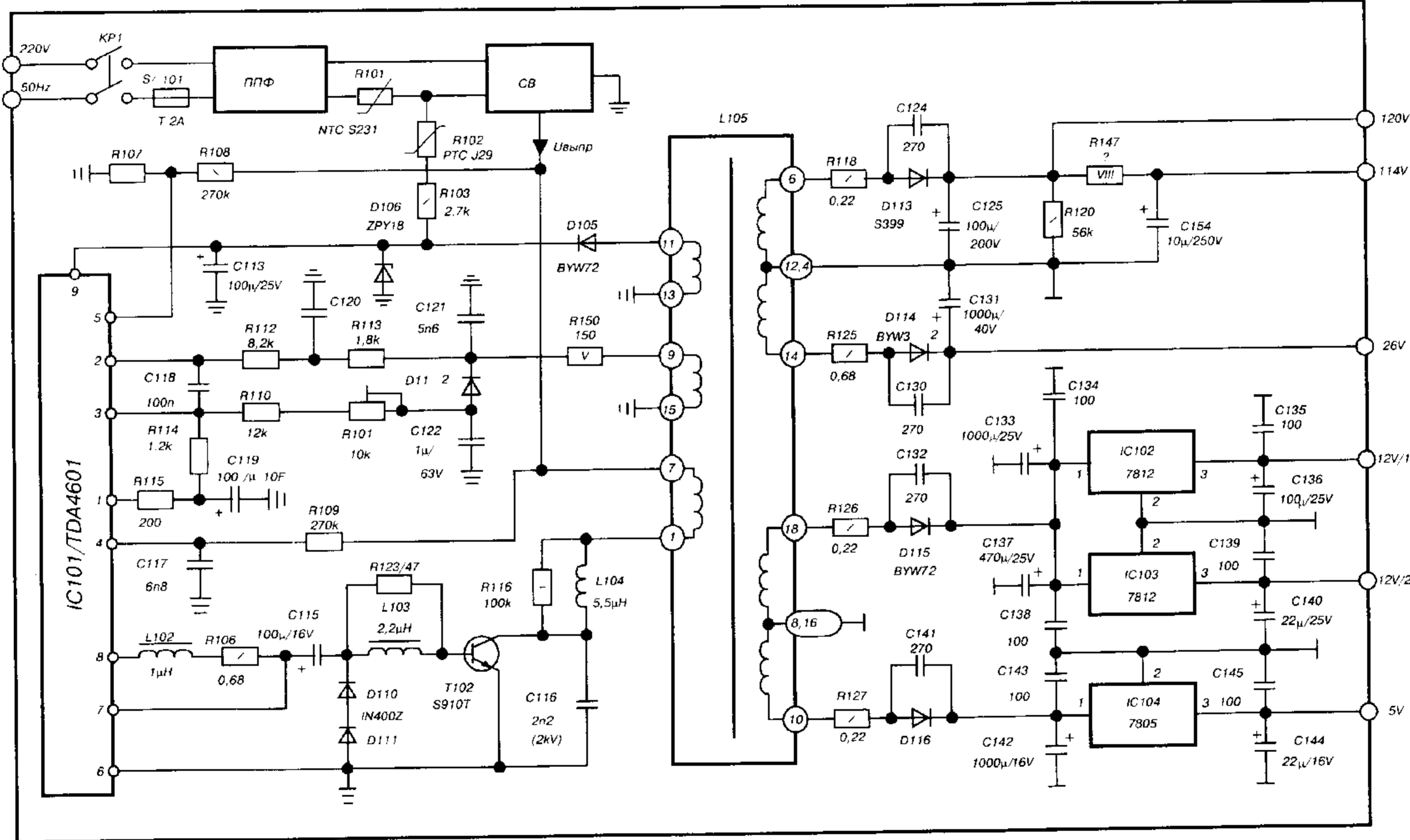
Схема блока питания телевизора WALTHAM TS-3341 Импульсный источник питания телевизора "WALTHAM TS3341"
