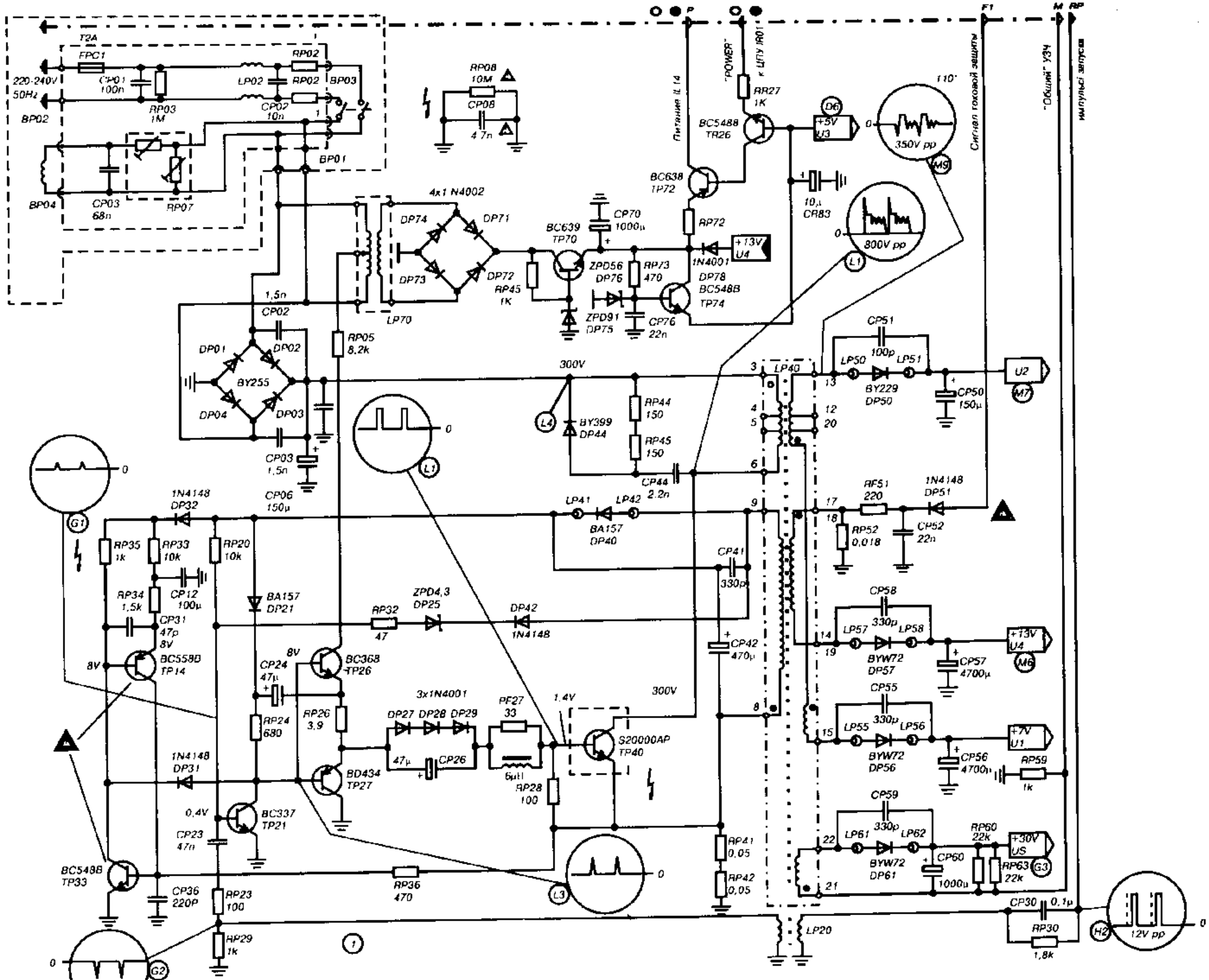
Схема блока питания телевизора WALTHAM TS-3350
