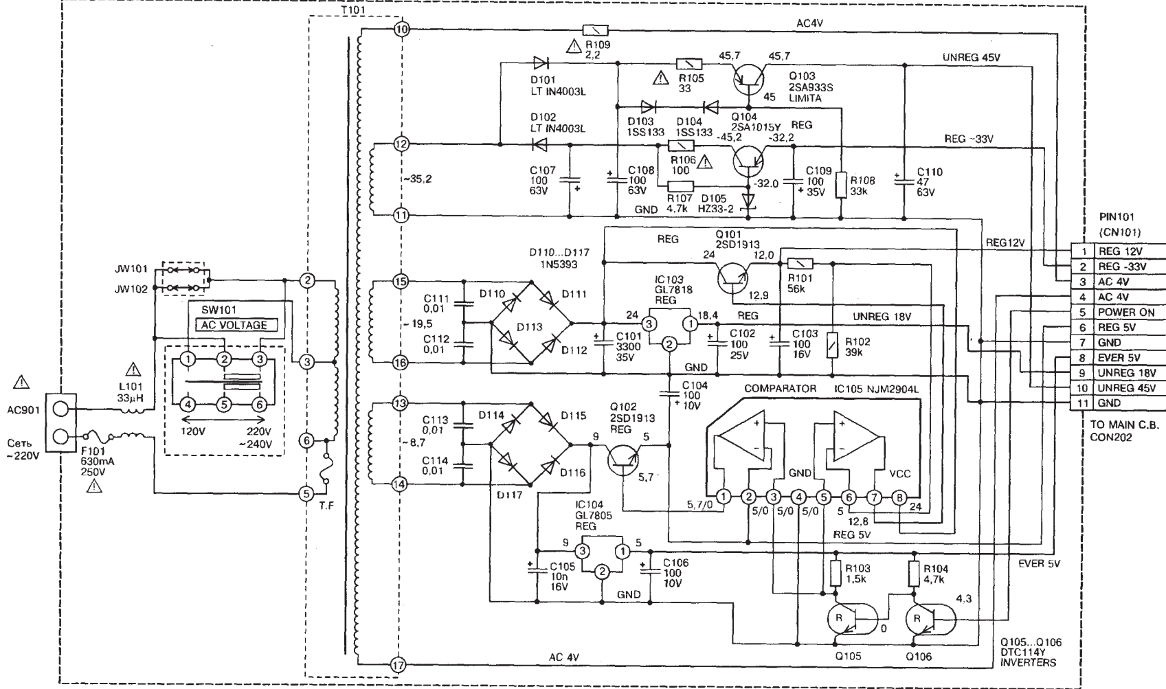
Схема блока питания видеоманитофона AIWA HV-DK925/975/G100/110/150
