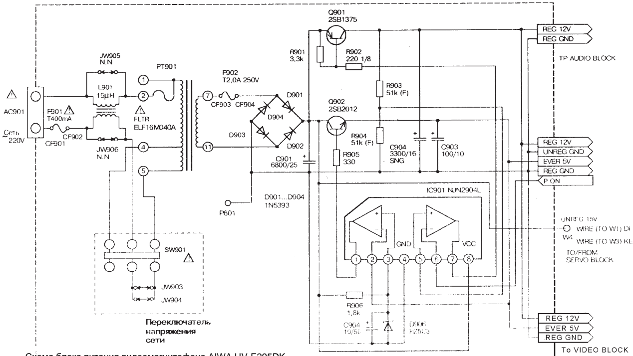
Схема блока питания видеомагнитофона AIWA HV-E295DK
