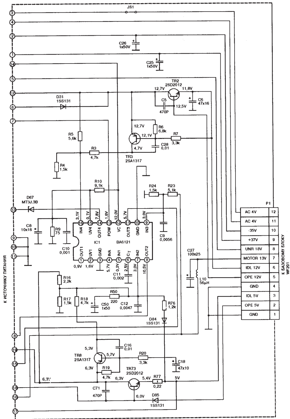
Схема блока питания видеомэгнофона AKAI VS-G44EOH-V, VS-G45EOG-V
