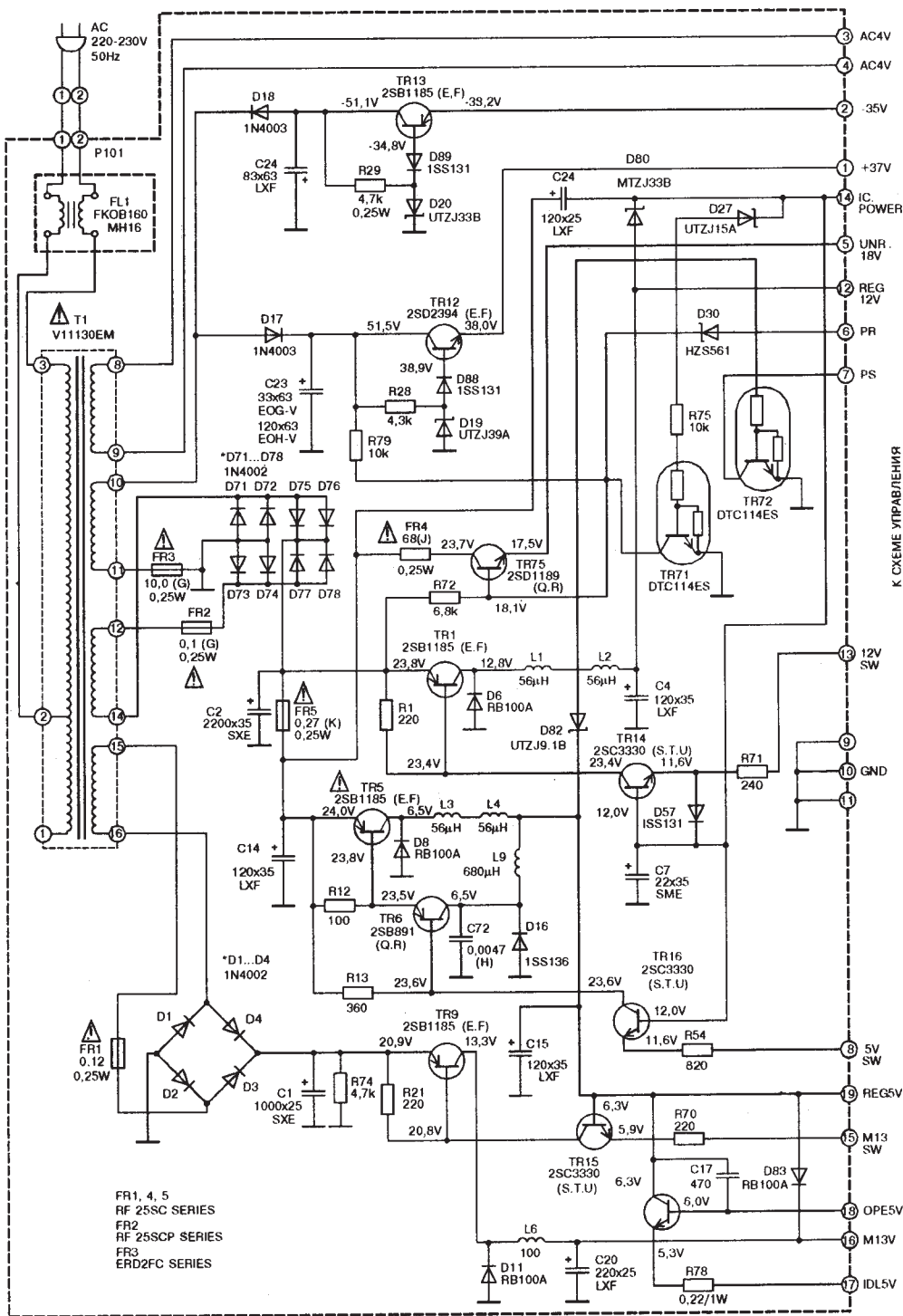
Принципиальная схема трансформаторного блока источника питания видеомэагнитофонов VS-G44EOH-V/G45EOG-V
