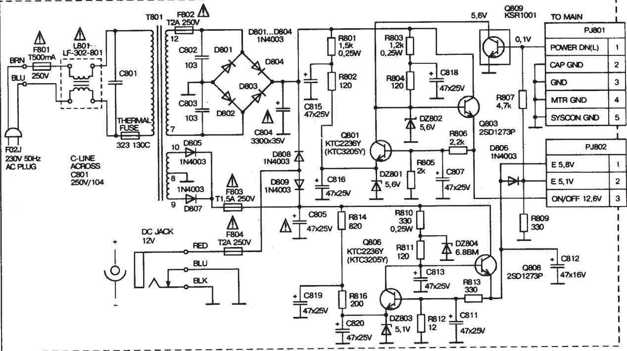
Схема блока питания видеомэгнофона DAEWOO DVR-1181D Принципиальная схема источника питания видеомэгнофонов DVR-1181D фирмы DAEWOO и VC-R14EMK фирмы ELEKTA.
