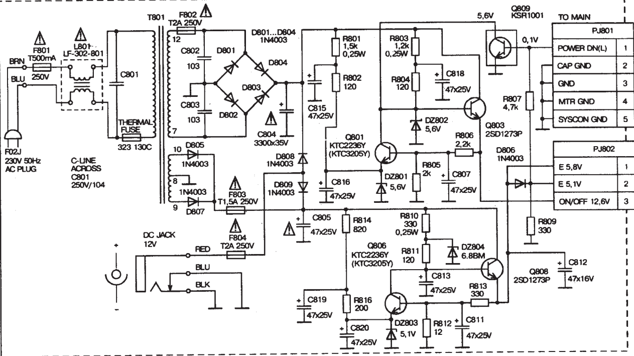
Схема блока питания видеомэагнитофона ELEKTA VC-R14 EMK Принципиальная схема источника питания видеомэагнитофонов DVR-1181D фирмы DAEWOO и VC-R14EMK фирмы ELEKTA.
