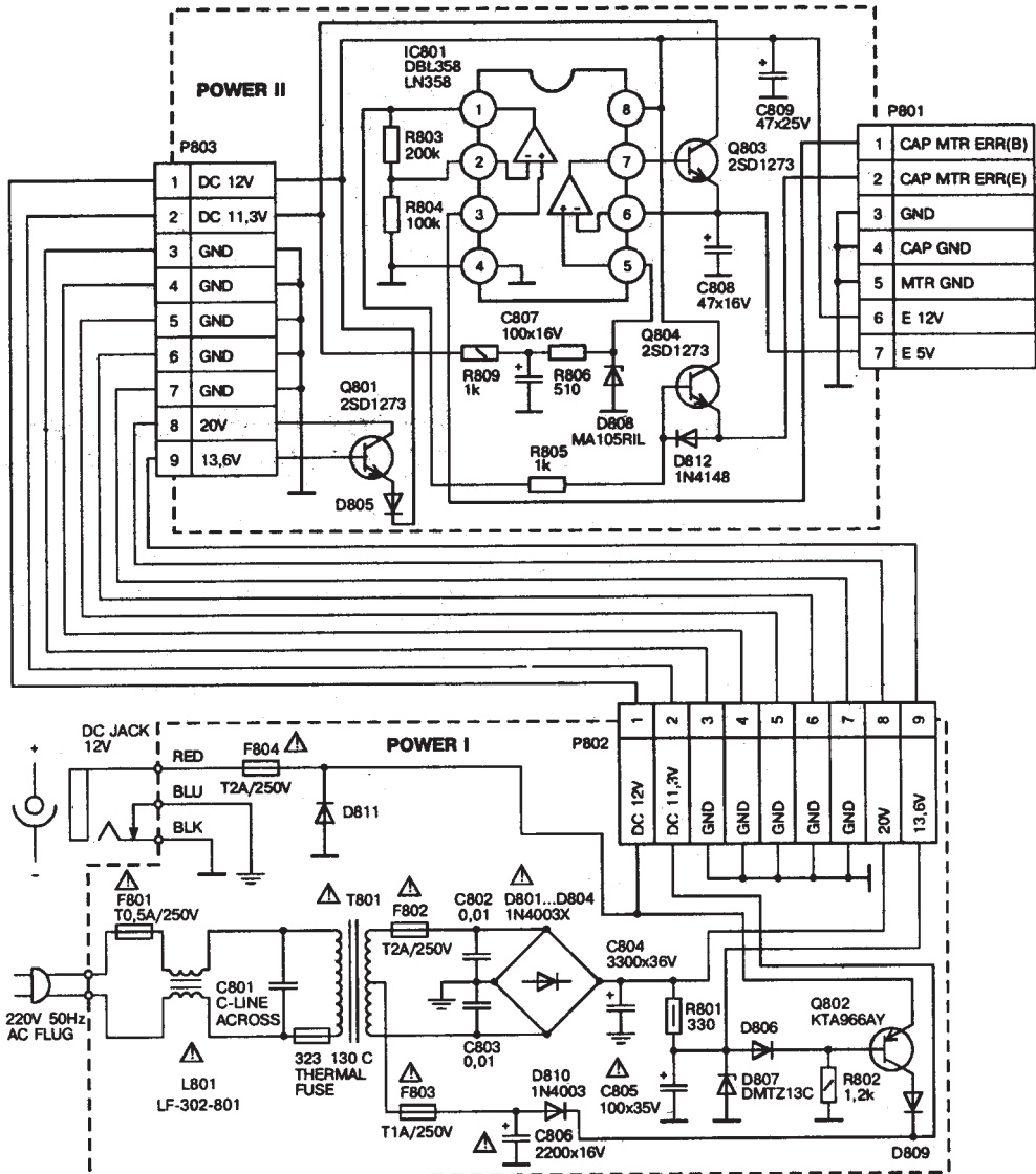
Схема блока питания видеомагнитофона ELEKTA VCP-5950 EMK
