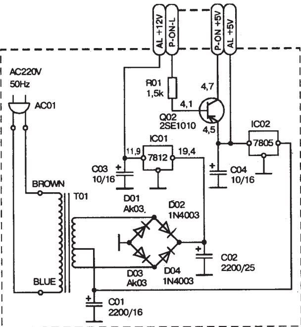
Схема блока питания видеомagnитoфона FUNAI VIP-3000HC/5000HC, VIP-8000K
