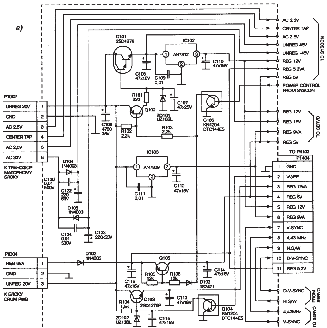
Схема блока питания видеомагнитофона GOLDSTAR GHV-1245W/1246W
