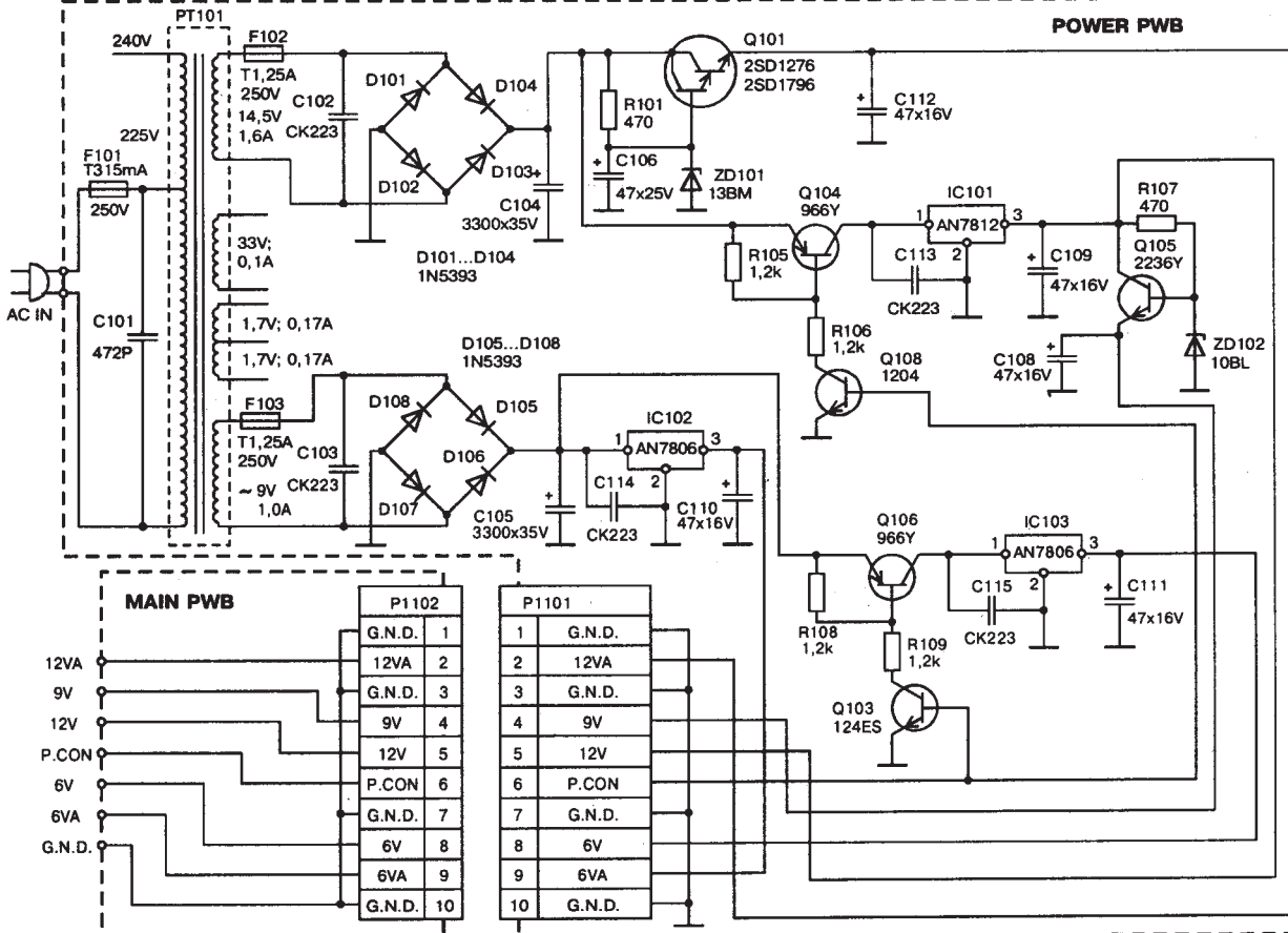
Схема блока питания видеомагнитофона GOLDSTAR VCP-R1010P/R1110P
