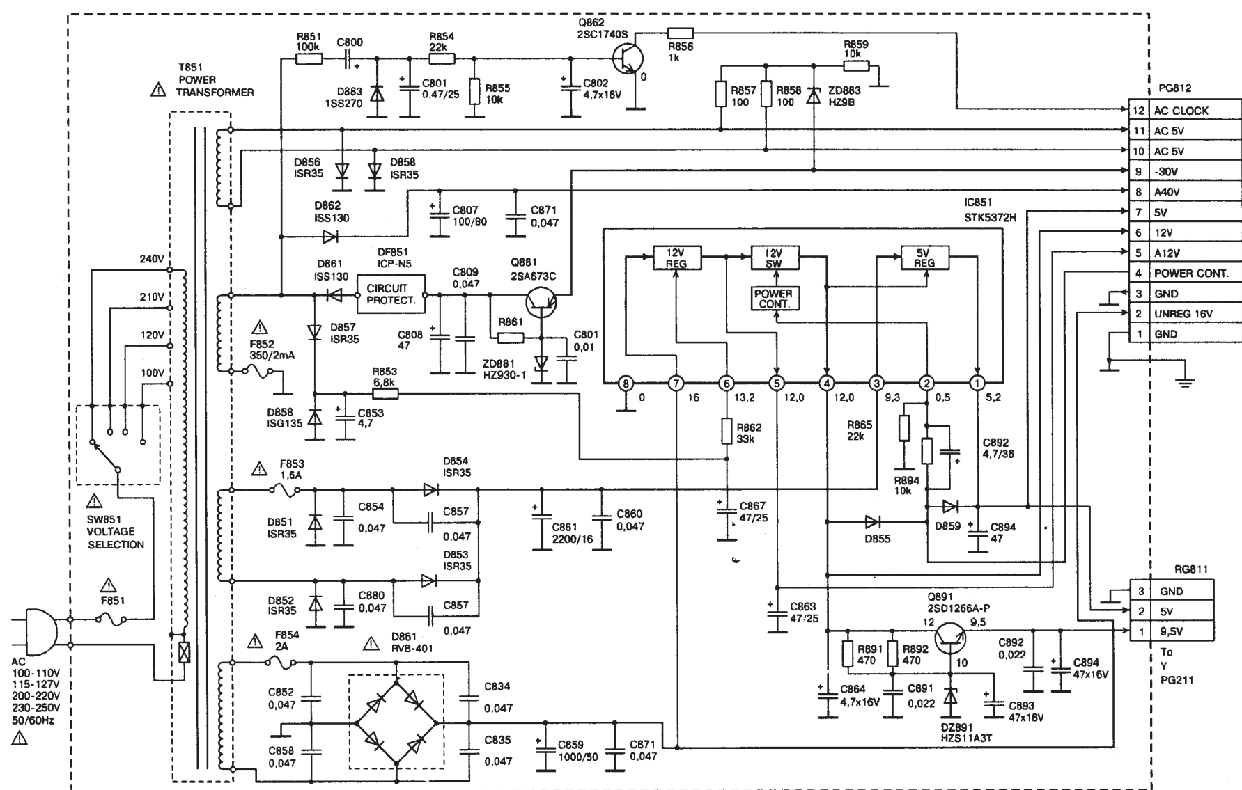
Схема блока питания видеомэагнитофона HITACHI VT-498EM
