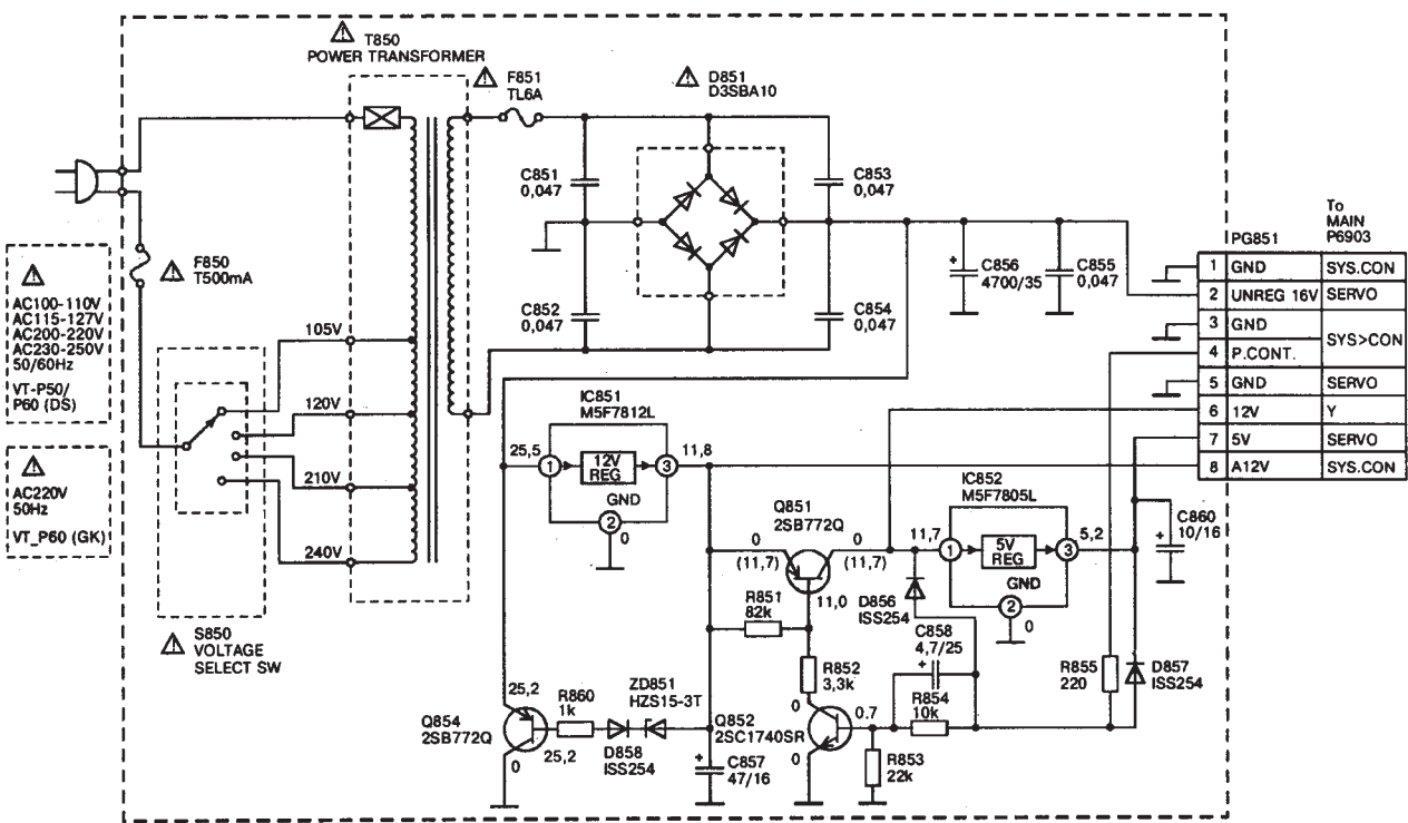
Схема блока питания видеомагнитофона HITACHI VT-P50/P60
