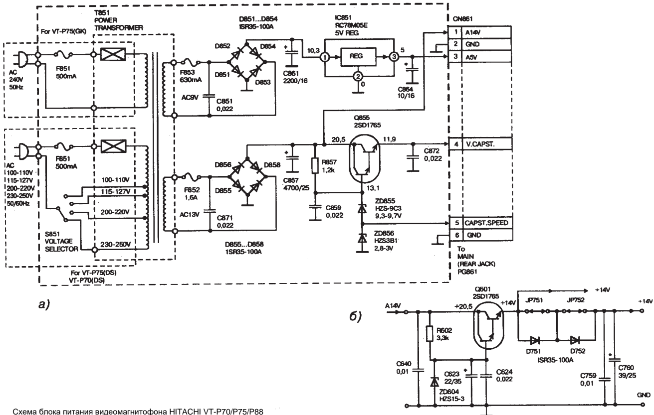
Схема блока питания видеомагнитофона HITACHI VT-P70/P75/P88
