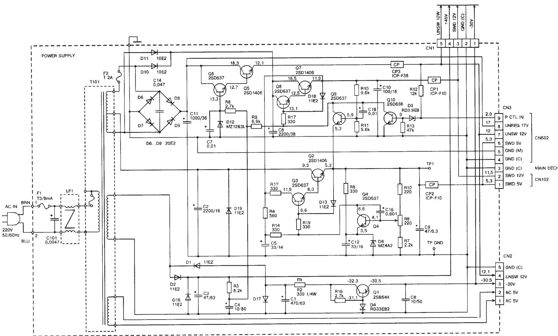
Схема блока питания видеомэагнитофона JVC HR-D150E
