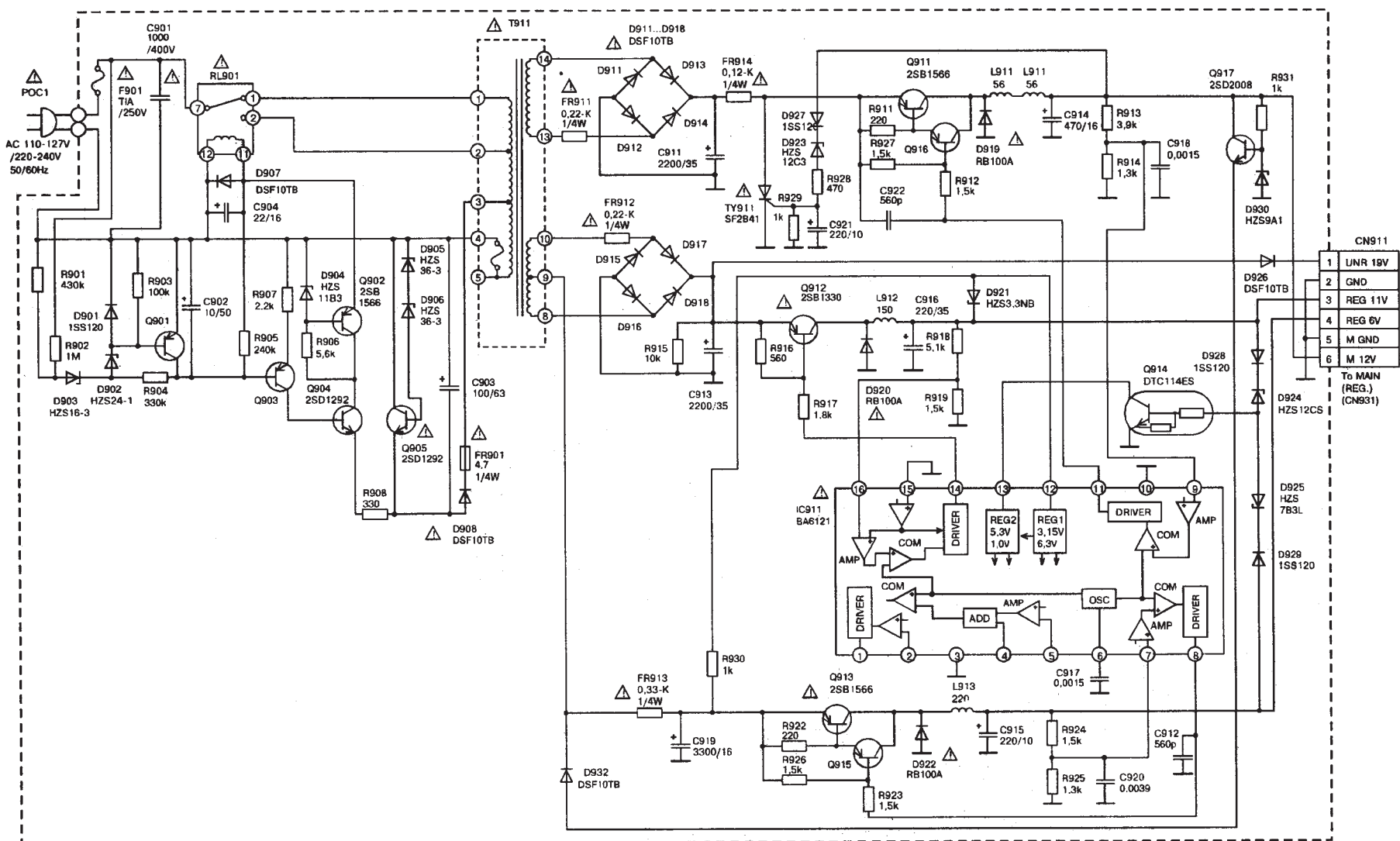
Схема блока питания видеомэгнофона JVC HR-P29A/P78K
