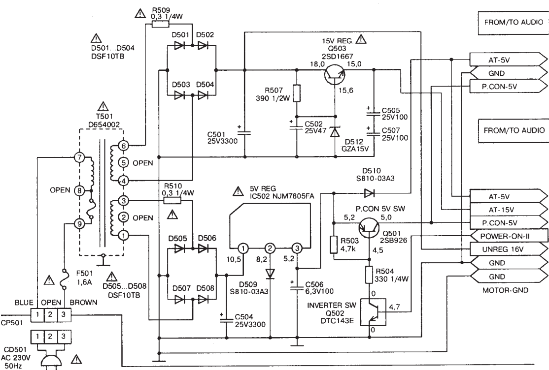
Схема блока питания видеоманитофона ORION VP-388
