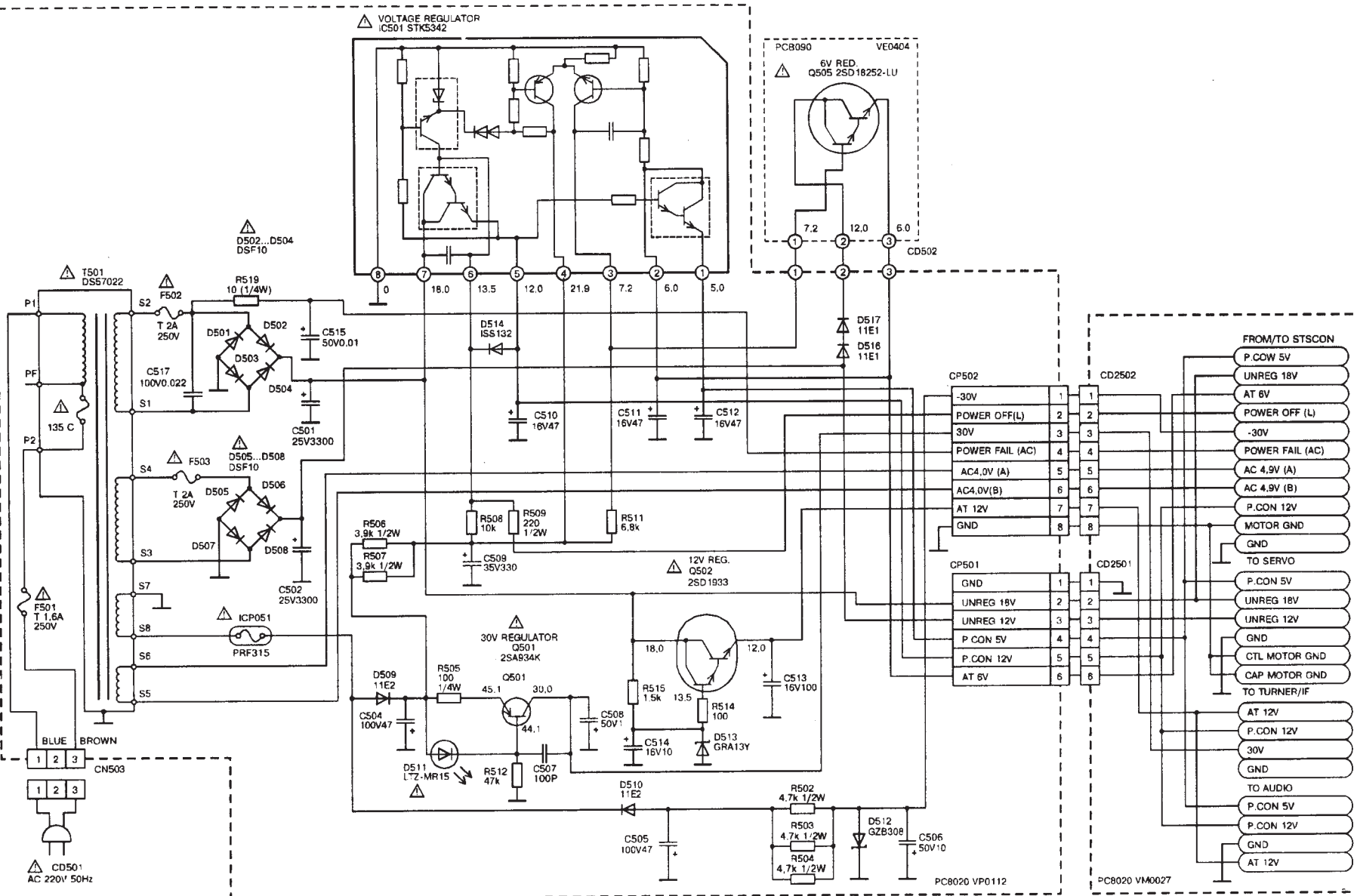
Схема блока питания видеомэагнитофона ОТАКЕ VCR-555
