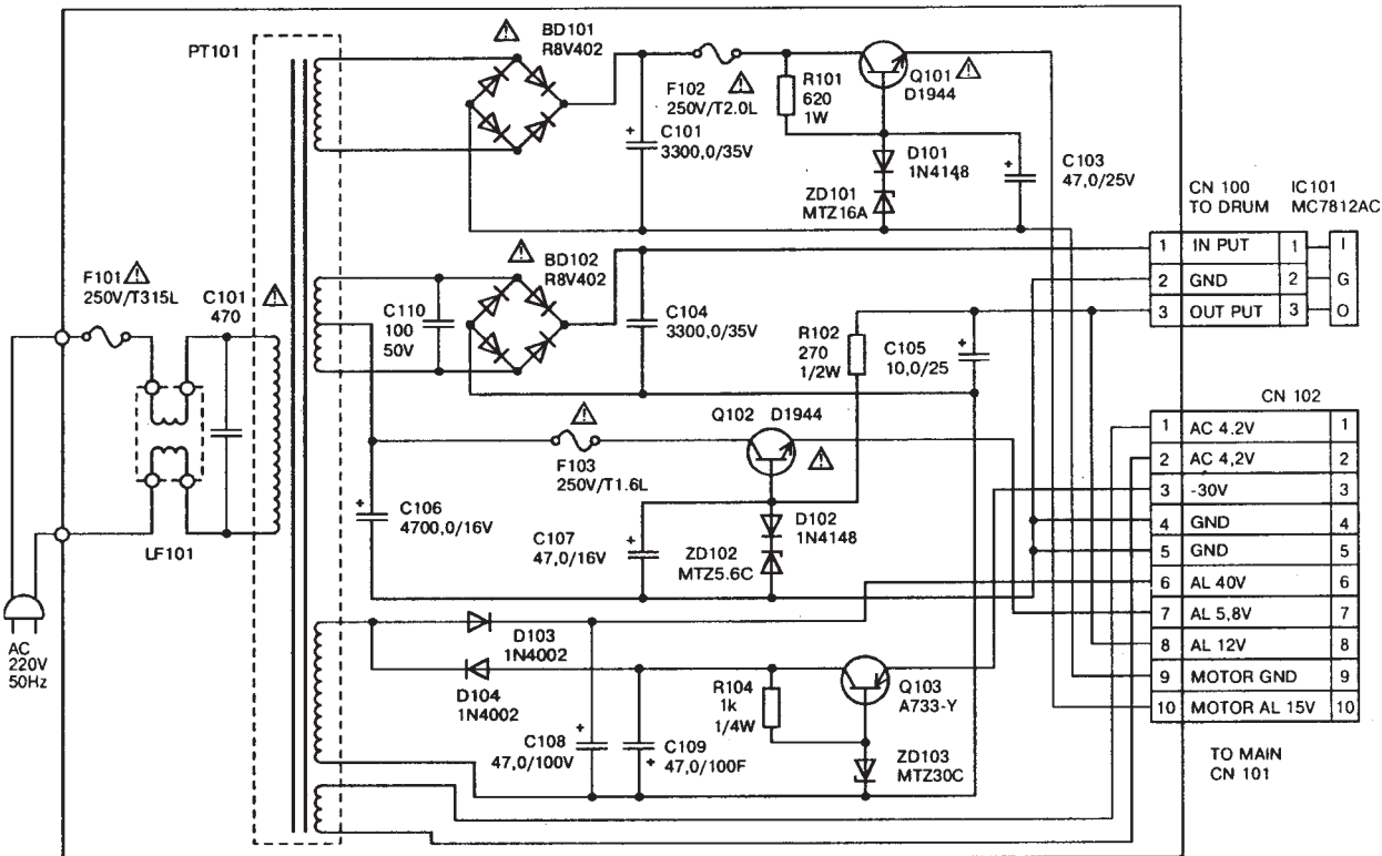
Схема блока питания видеомэагнитофона SAMSUNG VK-1230/1260/1560
