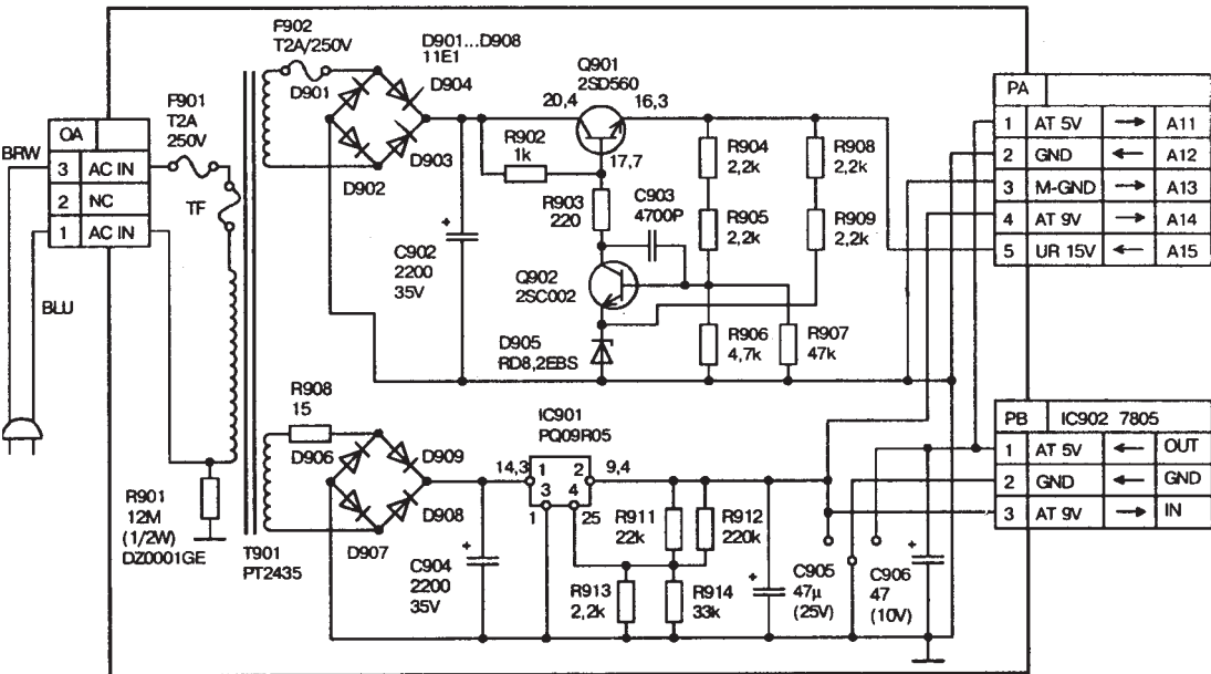
Схема блока питания видеомэагнитофона SHARP VC-6V3DR
