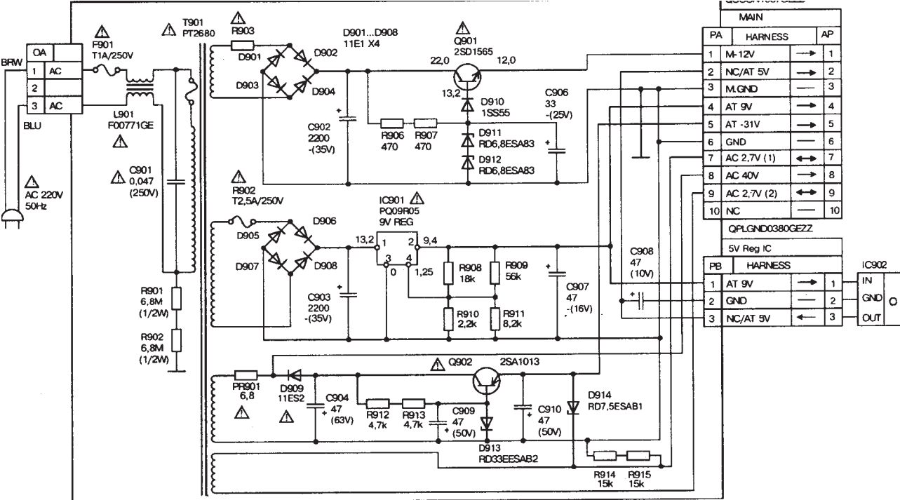
Схема блока питания видеомэагнитофона SHARP VC-A30B
