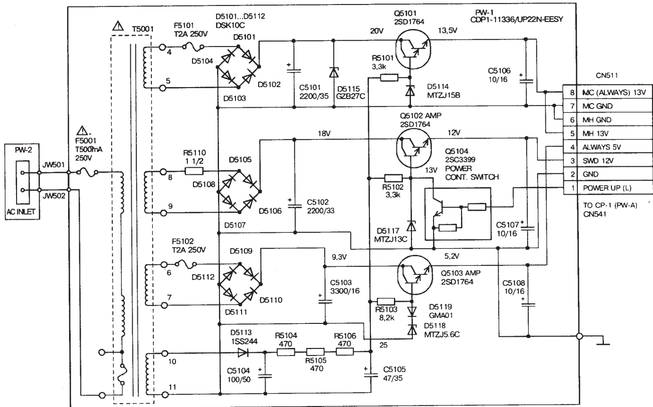
Схема блока питания видеомэгнофона SONY SLV-P116EE Принципиальная схема источника питания видеомэгнофона SLV-P116EE фирмы SONY.
