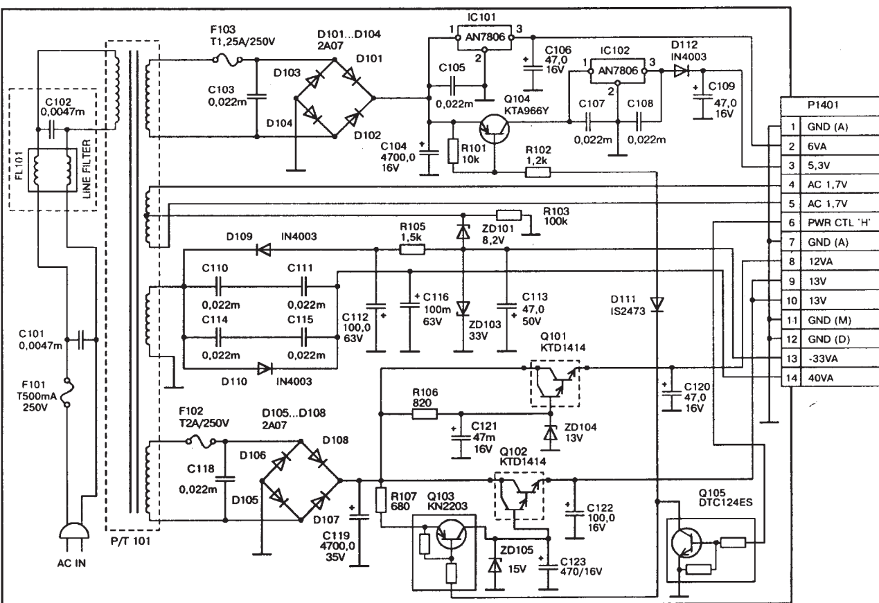
Схема блока питания видеоматрицы SUPRA SV-T21 Принципиальная схема источника питания видеоматрицы SV-T21 фирмы SUPRA.
