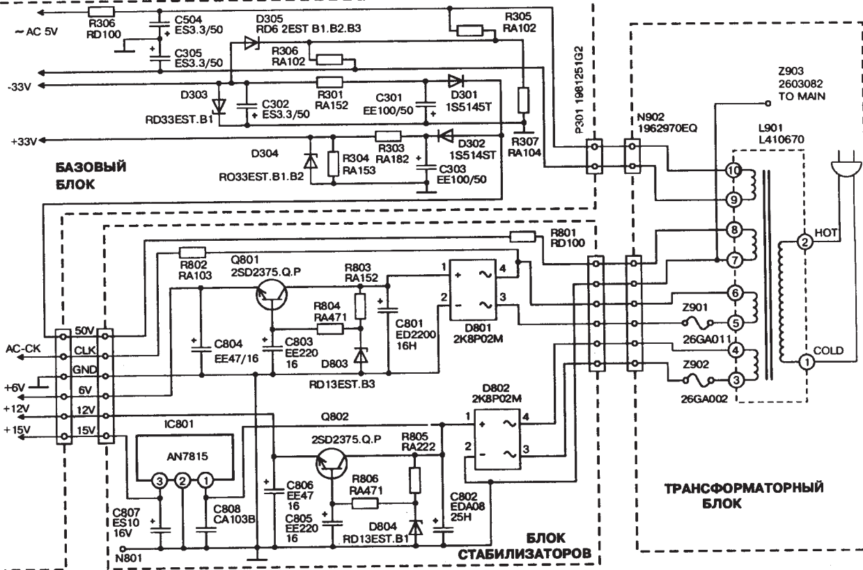
Схема блока питания видеомagniфона SUPRA SV-T25
